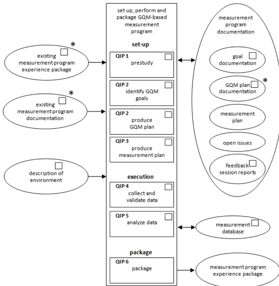
Figura 3-14: Vista funcional del proceso general de GQM (tomado de [Gresse, y otros, 1995]).
