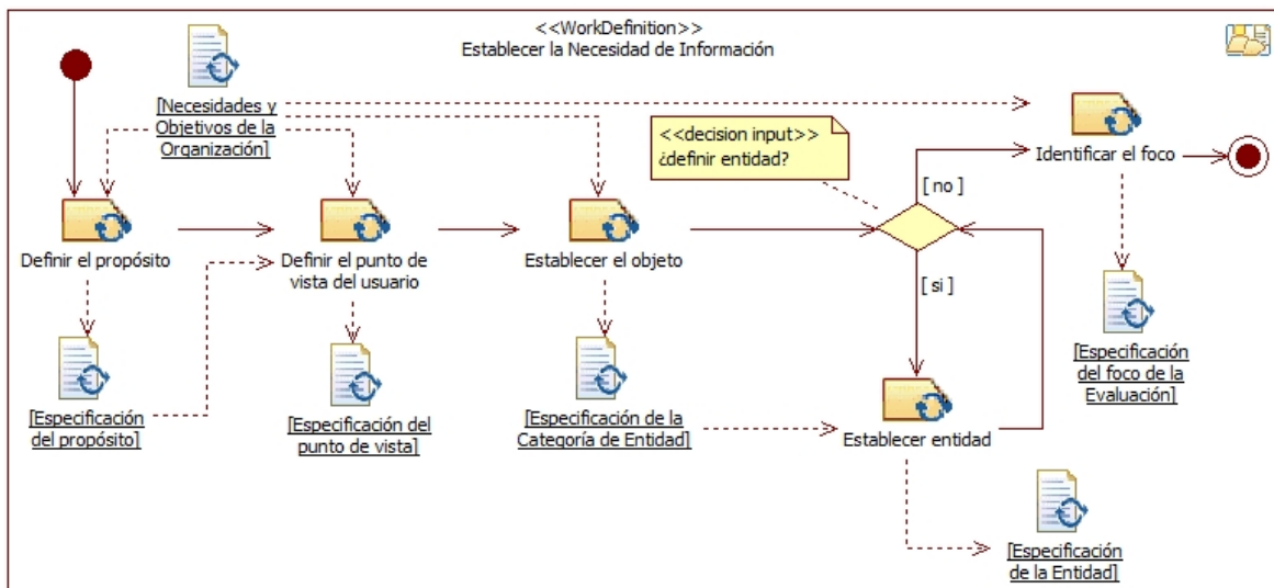
Figura 4-5: Vista funcional y de comportamiento de la actividad Establecer la Necesidad de Información .
