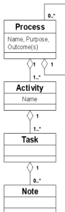
Figura 3-17: Constructores de proceso según ISO/IEC 12207/15288 (tomado de [ISO/IEC, 2004]).
