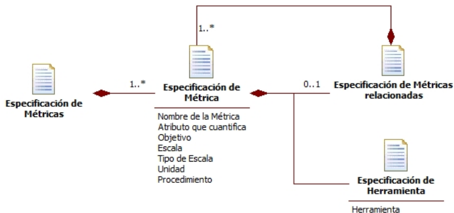
Figura 4-31: Composición del artefacto Especificación de Métricas .
