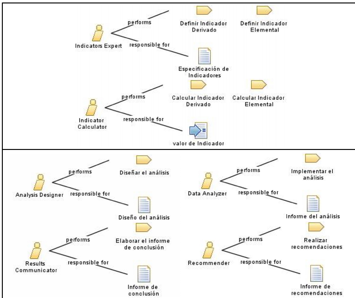
Figura 4-29: Roles de las actividades A4, A5 y A6, asociados a las tareas que ejecutan y los productos de trabajo por los cuales son responsables.
