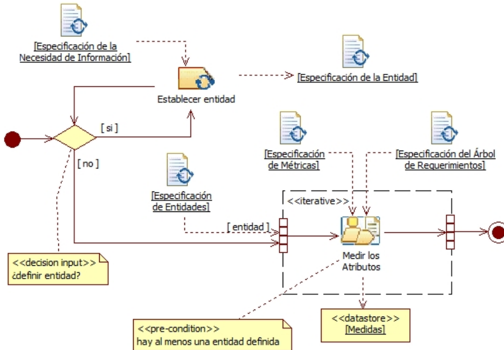
Figura 4-14: Actividad Implementar la Medición .
