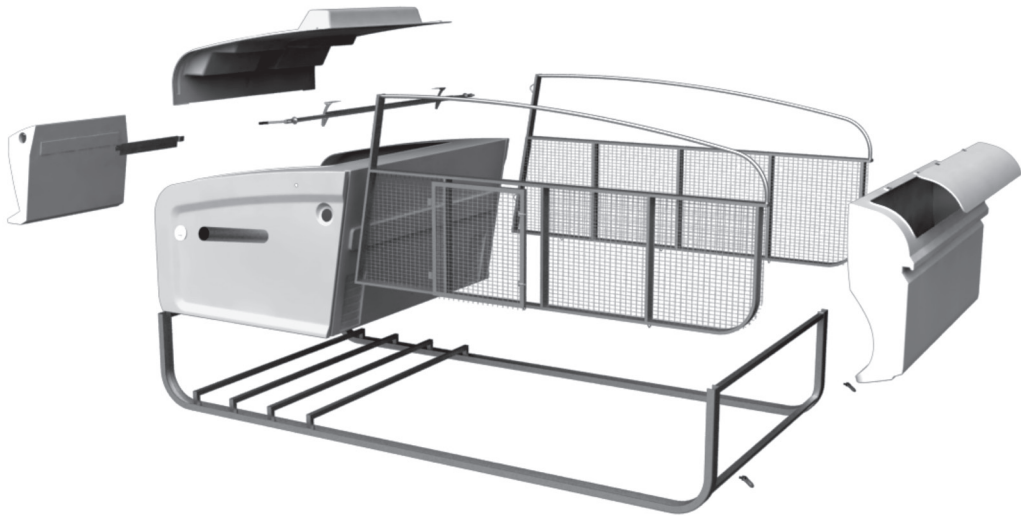
FIGURA 3. Despiece
