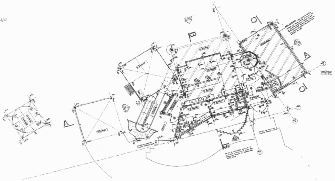
Planta nivel + 2.75
