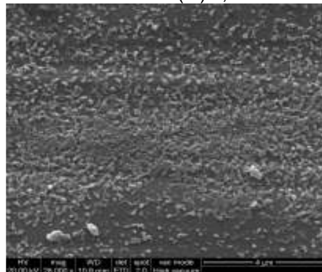
Figura 3.4. Morfología de la película protectora sobre el acero SAE 1010 en contacto con nitrato de cerio (III) 4,60 \times 10^{-4} M
