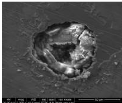
Figura 3.6. Morfología de una picadura de la película protectora sobre el acero SAE 1010 en contacto con nitrato de cerio (III) 3,40 \times 10^{-4} M
