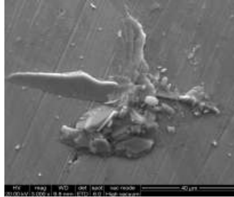
Figura 3.2. Acumulaciones de óxido de cerio (III) sobre la película protectora del acero SAE 1010 con nitrato de cerio (III) 1,15 \times 10^{-4} M
