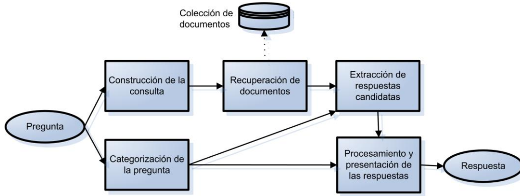
Figura 2. Arquitectura básica para la búsqueda de respuestas
