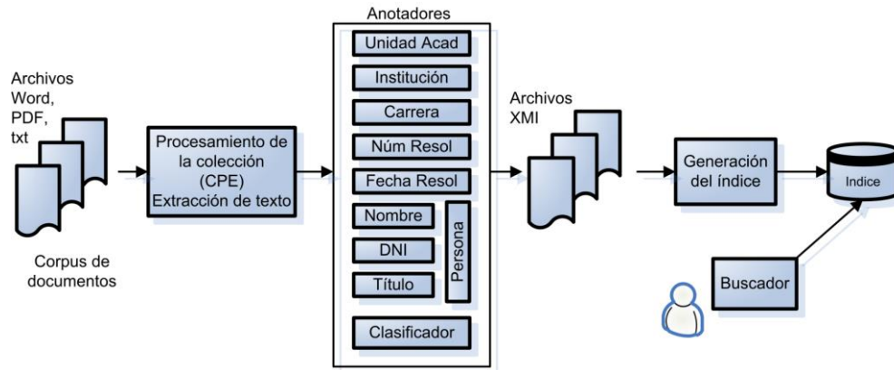
Figura 1. Arquitectura del sistema de gestión de información no estructurada.
