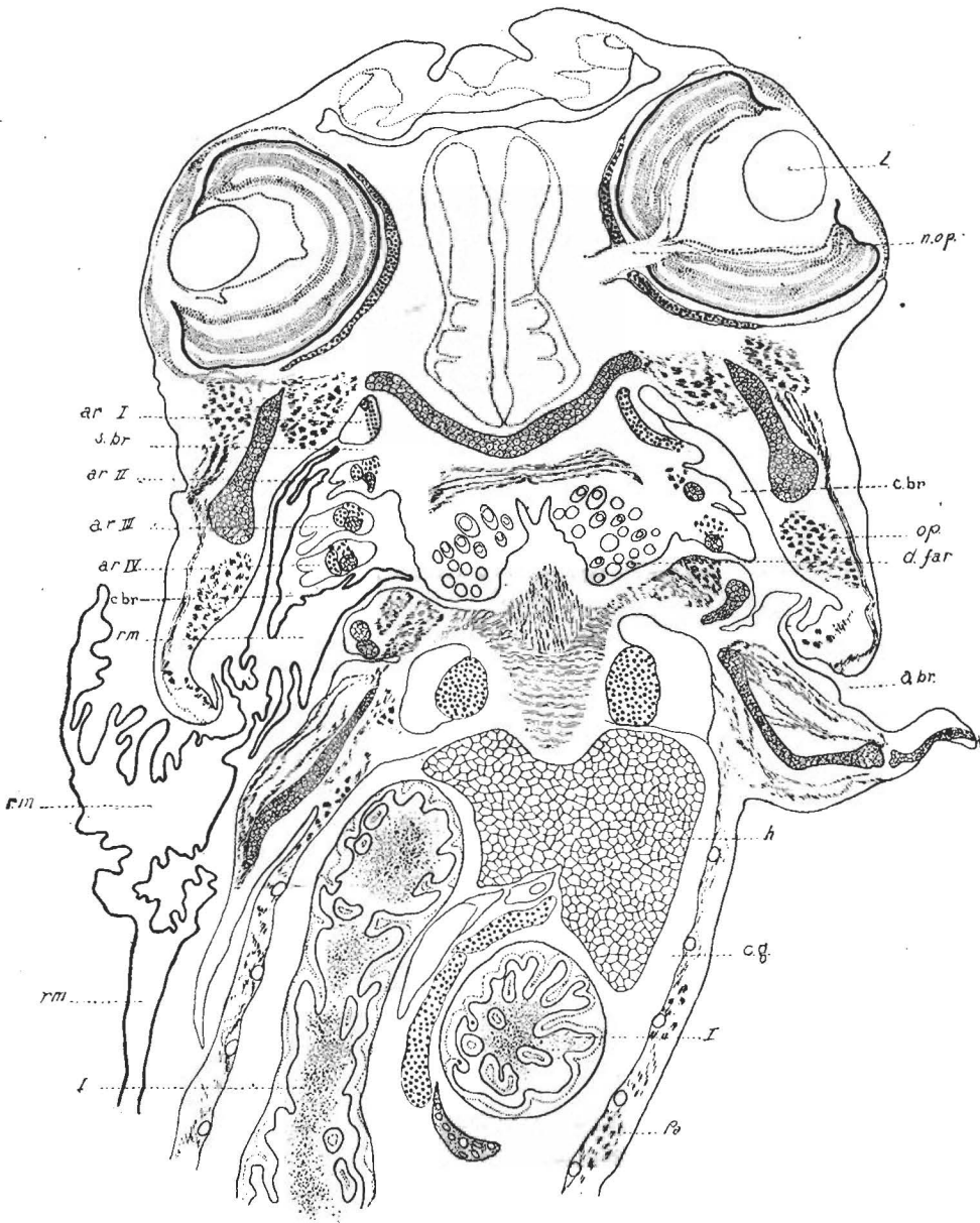
Fig. 2. — Corte longitudinal horizontal por un embrión de Jenynsia lineata . ar. I, II, III, IV, V, arcos branquiales; a. br, apertura branquial; c. br, cavidad branquial; c. g., cavidad general; d. far, dientes faringeos; h, hígado; I, intestino; L, lente; n. op., nervio óptico; op., opérculo; pa, pared del cuerpo; rm, repliegue ovarial materno (× 20)
