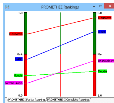
Figura 5: Resultado: Rankings PROMETHEE I. Visual PROMETHEE.
