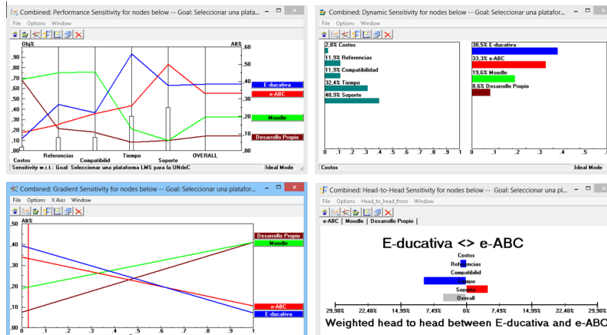
Figura 3: Gráficos de sensibilidad de Expert Choice.
