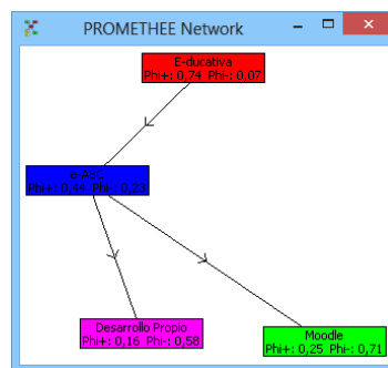
Figura 8: Resultado: Network. Visual PROMETHEE.
