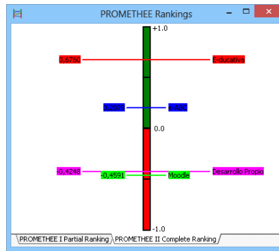
Figura 6: Resultado: Rankings PROMETHEE II. Visual PROMETHEE.
