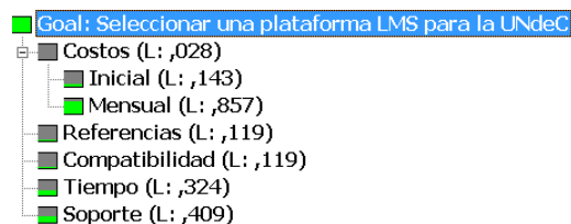
Figura 1: Estructura jerárquica de criterios y prioridades.
