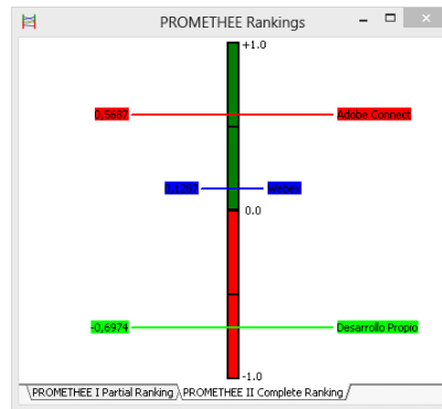
Figura 9: Resultado: Rankings PROMETHEE II. Visual PROMETHEE.
