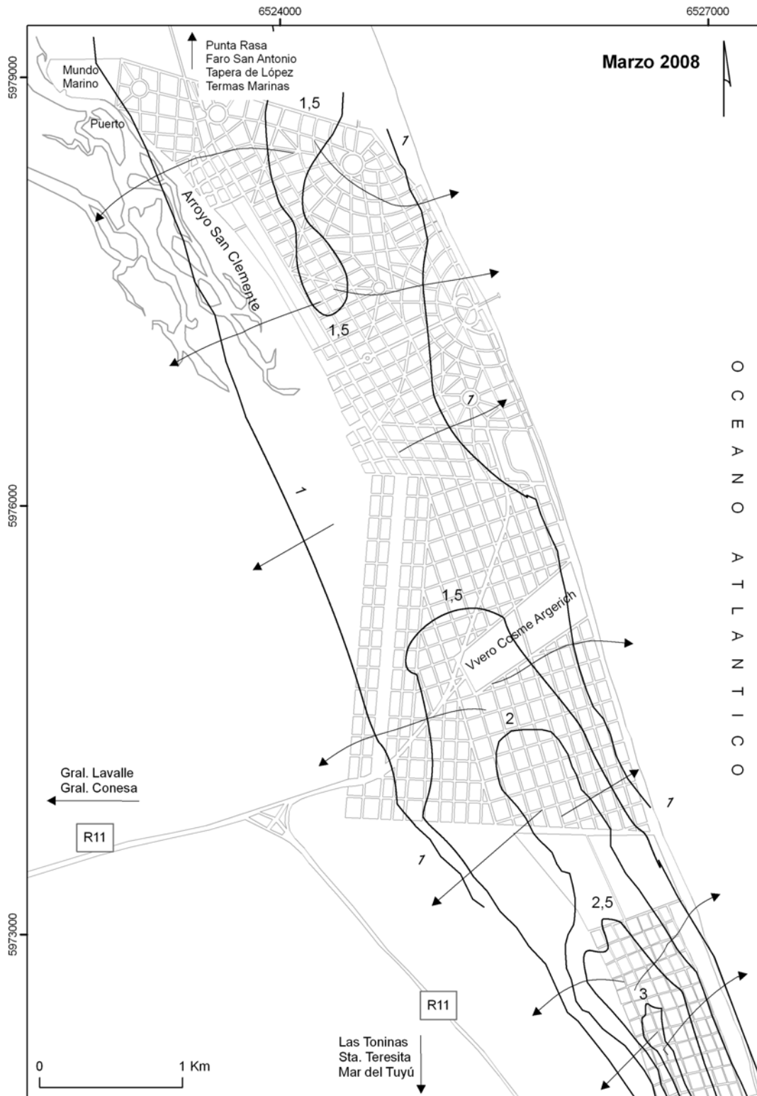
Figura 3. Mapa de flujo subterráneo para marzo de 2008 (curvas en m s.n.m.)
