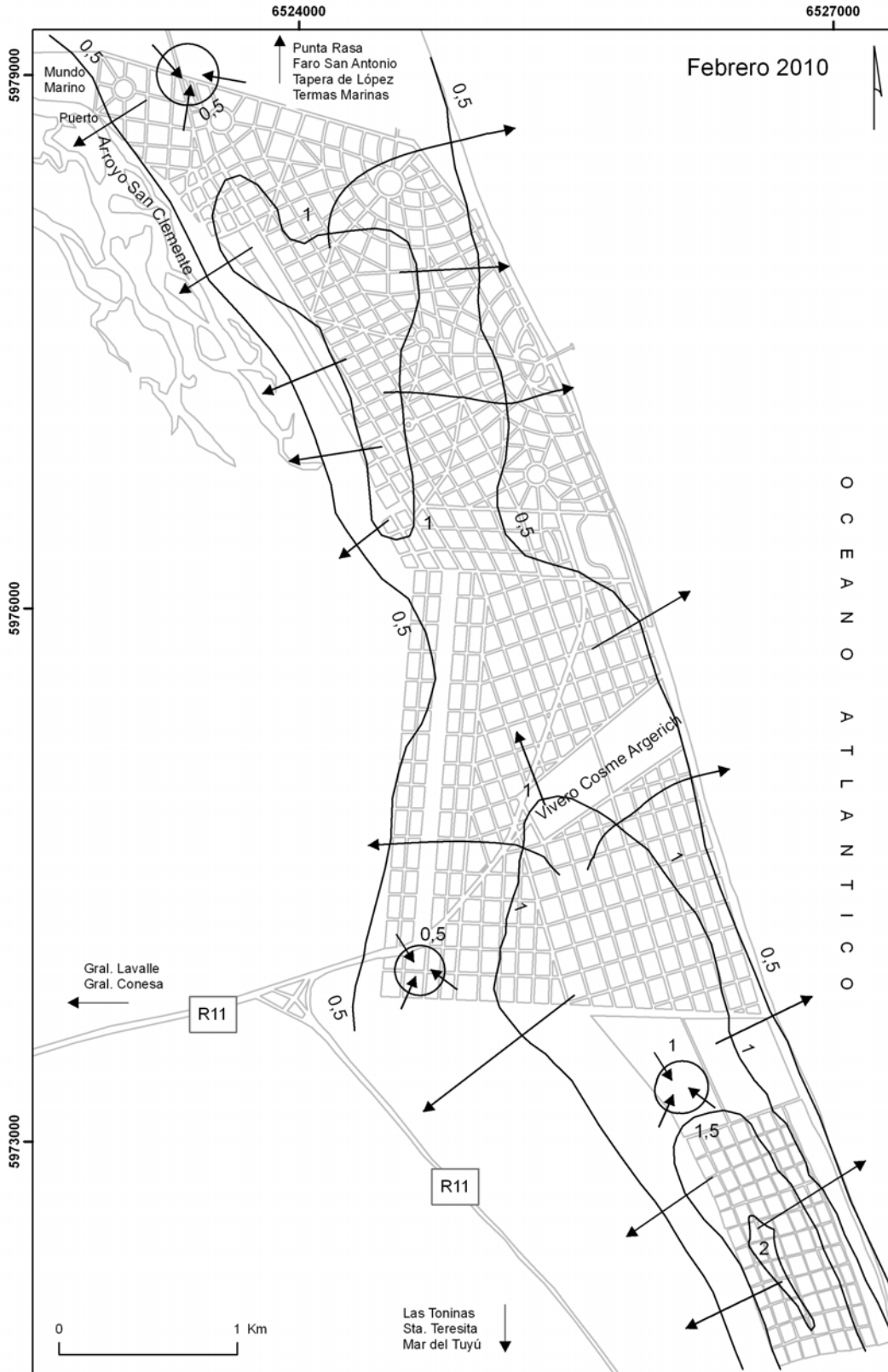
Figura 24. Mapa de flujo subterráneo para febrero de 2010 (curvas en m s.n.m.)
