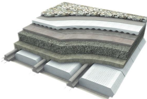
Fig. 17- Imagen 3D cubierta de viguetas invertida
