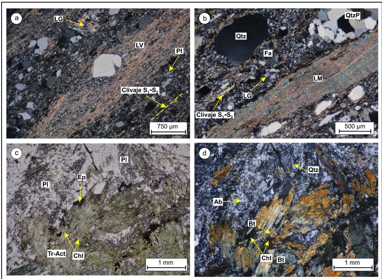
Figura 4.21. Fotomicrografías de los metaconglomerados de la litofacies verde grisácea y del filón capa en el área del arroyo Pajalta. (a) y (b) Luz transmitida y nicoles cruzados. (c) y (d) Fotomicrografías de la misma imagen tomada con luz transmitida y nicoles paralelos, y con luz transmitida y nicoles cruzados, respectivamente. Minerales metamórficos: Ab (albita), Bt (biotita), Chl (clorita), Ep (epidoto), Tr-Act (tremolita-actinolita). Granos detríticos: Fa (feldespato alcalino), LG (líticos ígneos graníticos), LM (filita-pizarra), LV (lítico volcánico), PI (plagioclasa), Qtz (cuarzo), QtzP (cuarzo policristalino). (a) y (b) Metaconglomerado lítico con granos detríticos de cuarzo, feldespato alcalino, plagioclasa, y fragmentos líticos metamórficos (cuarzo policristalino y filita) e ígneos (microgranítico). Los detritos están rodeados de una matriz recristalizada que contiene la paragénesis mineral de biotita + muscovita + clorita + epidoto + cuarzo + albita + turmalina. El fragmento lítico volcánico en (a) es una fenoriotita que muestra un fenocristal de cuarzo bipiramidal engolfado. El feldespato alcalino indicado en (b) es perítico y presenta sombras de deformación y strain cap . Observar los bordes de grano recto y uniones triples (recristalización estática) presentes en el cuarzo que compone la matriz recristalizada (a) y (b) y los granos detríticos de cuarzo policristalino (b). Los granos detríticos de cuarzo que se encuentran abajo a la derecha en (b) están aplanados y estirados según el clivaje S_1-S_2 . (c) y (d) Metagabbro/diorita de la zona central del filón capa. La plagioclasa conserva su forma relíctica tabular ígnea pero está reemplazada fundamentalmente por epidoto + albita. Tremolita-actinolita + biotita marrón verdosa reemplazan al anfíbol ígneo. Observar al centro y arriba cuarzo y feldespato alcalino en un arreglo micrográfico probablemente de origen ígneo. La biotita marrón verdosa a su vez reemplaza parcialmente a la tremolita-actinolita.
