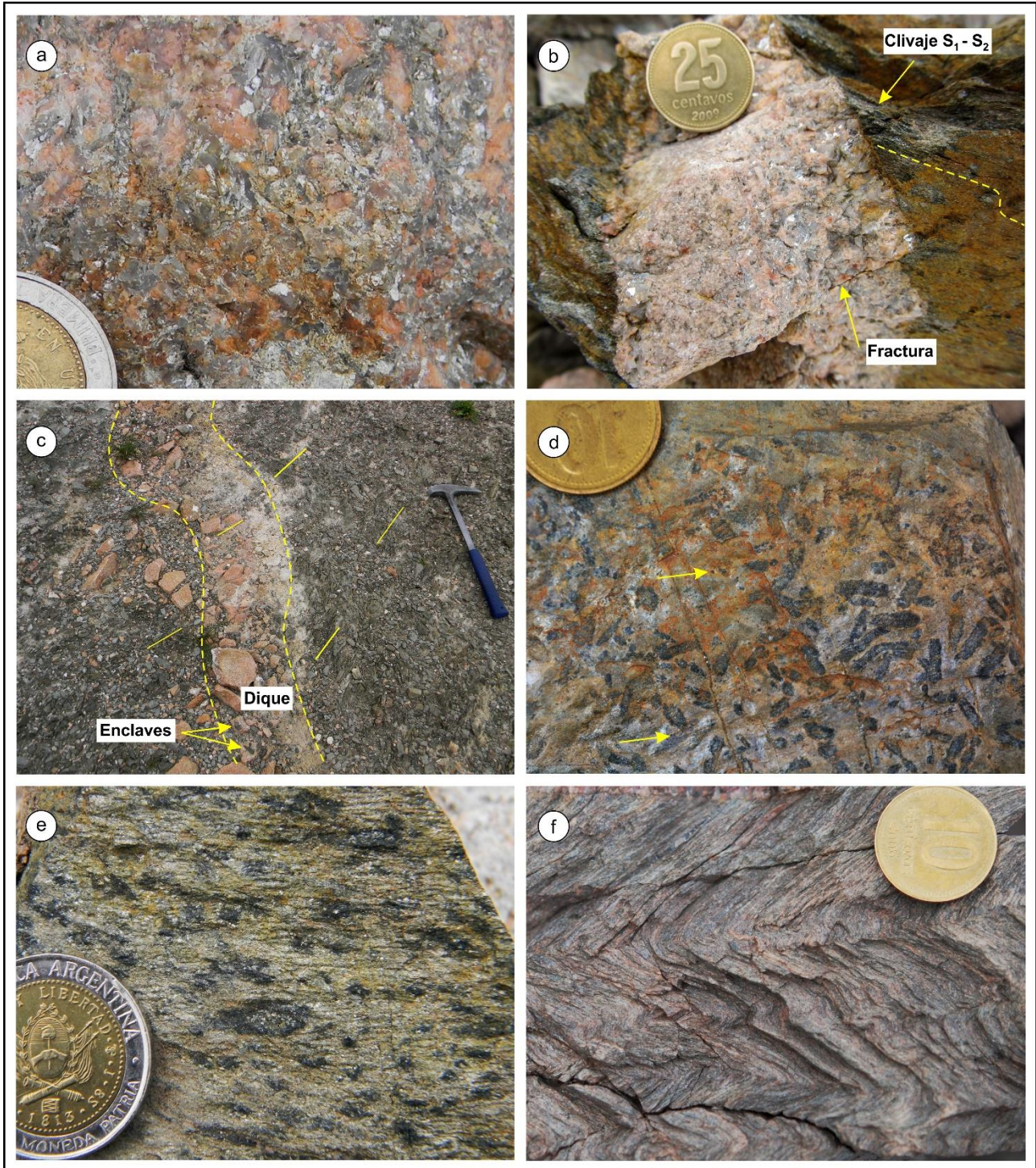
Figura 4.29. Características de los afloramientos de los granitos del Complejo Plutónico Punta Sierra y las metamorfitas de la Formación Nahuel Niyeu sobre la Ruta Nacional 23. (a) Aspecto de los leucogranitos muscovíticos de grano medio del plutón Valcheta. (b) Dique de leucogranito muscovítico cortando al clivaje S_1-S_2 de filitas de la litofacies verde grisácea. La roca de caja presenta evidencias de metamorfismo de contacto producida por la tonalita del Complejo Plutónico Navarrete del Pérmico (porfiroblastos de andalucita y biotita y crecimiento de las micas que forman S_1-S_2 ). El dique de leucogranito presenta bordes pegmatíticos. Un pliegue kink F_3 (línea punteada) que afecta a la filita se transfiere como una fractura al dique de leucogranito. (c) Dique de leucogranito muscovítico y filitas con metamorfismo de contacto. Ambos están afectados por pliegue F_3 . Las líneas punteadas indican los contactos del dique. Líneas continuas indican el clivaje de crenulación S_3 , el cual se transfiere como fracturas en el dique. Los bordes del dique están muy cizallados. El dique presenta enclaves angulosos de las metamorfitas. La foto corresponde a la zona de charnela del pliegue F_3 . (d) Filita con porfiroblastos de andalucita crecidos en forma decusada sobre el clivaje S_1-S_2 . Los filosilicatos que forman el clivaje S_1-S_2 presentan crecimiento estático. Las flechas amarillas señalan porfiroblastos de biotita pequeños. Los porfiroblastos de andalucita están reemplazados por biotita y muscovita. La foto corresponde al flanco NO del pliegue F_3 del contacto oeste de la tonalita (Fig. 4.28). (e) Filita con porfiroblastos de andalucita y clivaje S_1-S_2 con crecimiento estático de los filosilicatos (muscovita + biotita) afectados por ejes de crenulación B_3 . Los (continúa)
