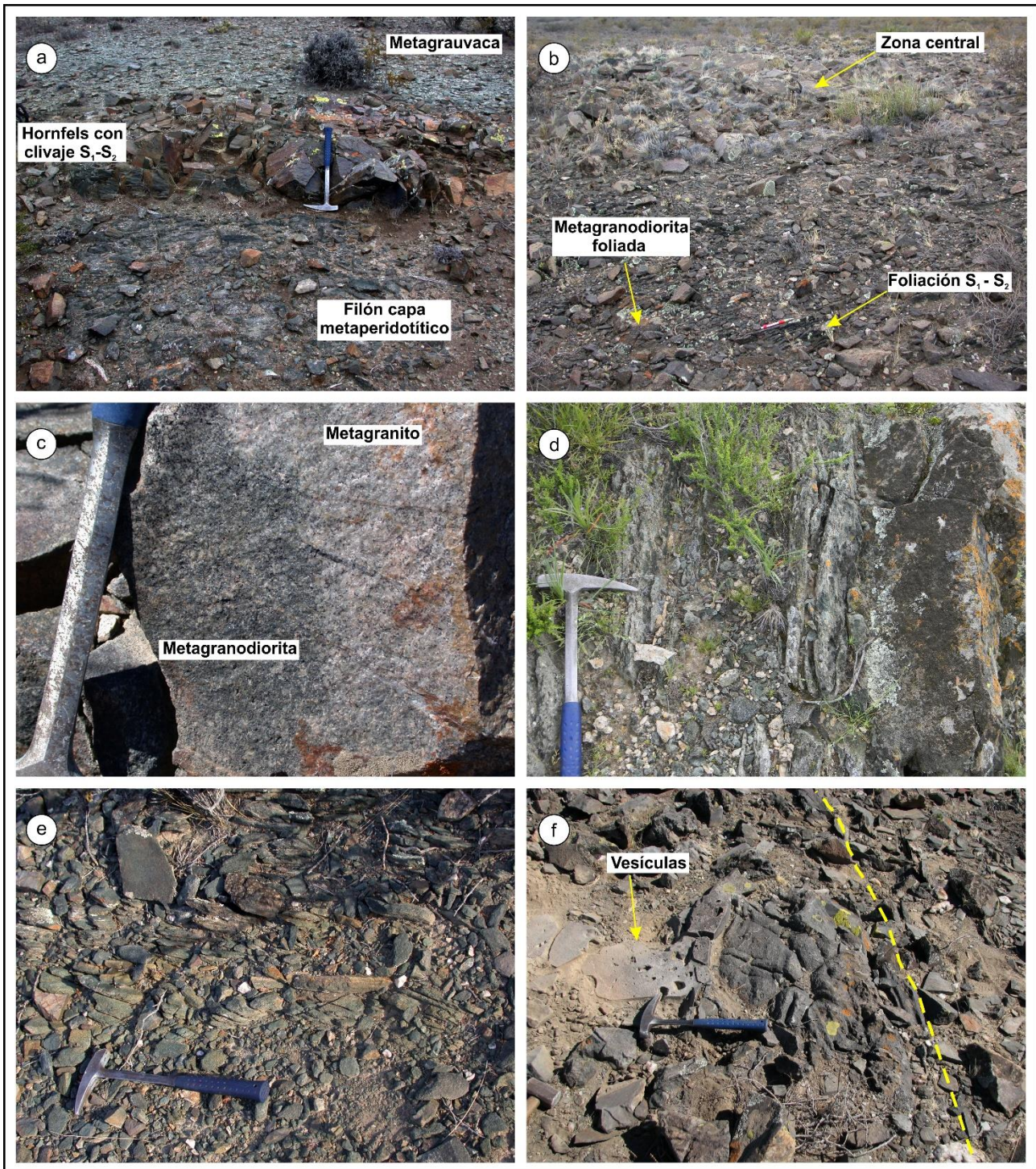
Figura 4.4. Características de los afloramientos de las rocas metaígneas de la Formación Nahuel Niyeu en Aguada Cecilio. (a) Contacto entre filón capa metaperidotítico y metagrauvascas de la litofacies verde grisácea mostrando un hornfels con desarrollo de clivaje S_1-S_2 . (b) Zona central y de borde del cuerpo principal de metagranodiorita de uno de los filones capa compuestos. La zona de borde presenta foliación penetrativa S_1-S_2 . (c) Contacto entre diferenciado metagranítico y metagranodiorita, ambas rocas preservan en forma relictica texturas ígneas granudas. De este metagranito se tomó la muestra V11-148. (d) Filón capa de metagabro/diorita parcialmente transformado en esquistos verde con una foliación penetrativa S_1-S_2 . La foto corresponde al contacto entre la zona central (no foliada) y de borde (foliada) de un filón capa simple. (e) Filón capa delgado transformado en esquistos verde con una foliación penetrativa S_1-S_2 . (f) Lava metaandesítica intercalada en las rocas metasedimentarias de la litofacies verde grisácea. La metaandesita muestra vesículas en el techo. La línea punteada indica el contacto concordante de la lava con la estratificación sedimentaria relictica S_0 . Observar en (a), (b), (d) y (e) que la foliación S_1-S_2 es la principal de la Formación Nahuel Niyeu.
