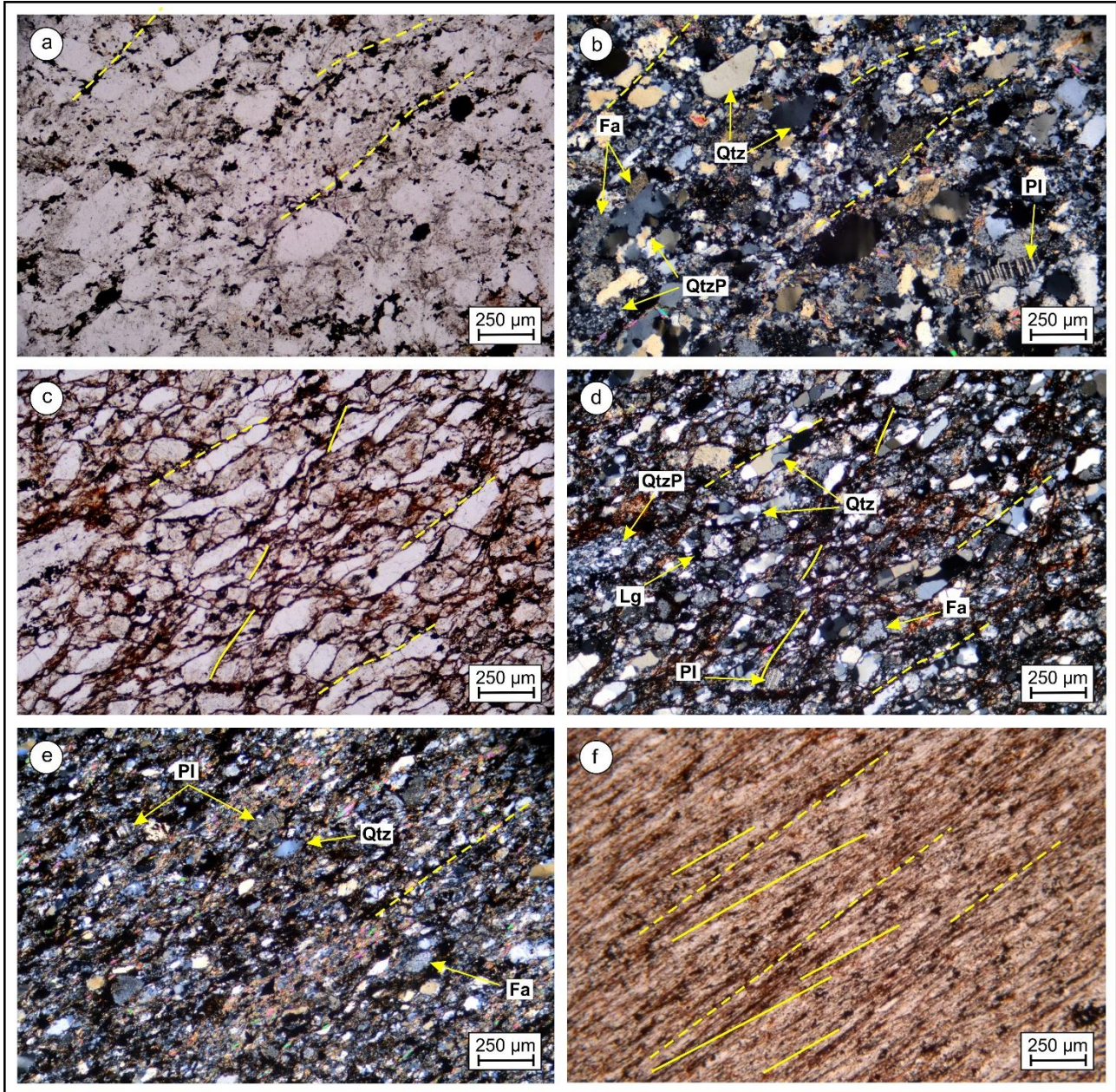
Figura 4.10. Fotomicrografías de las metasedimentitas de la litofacies roja en el área de Aguada Cecilio. (a) y (b) Fotomicrografías de la misma imagen tomada con luz transmitida y nicóles paralelos, y con luz transmitida y nicóles cruzados, respectivamente. (c) y (d) Ídem. (e) Fotomicrografía tomada con luz transmitida y nicóles cruzados. (f) Fotomicrografía tomada con luz transmitida y nicóles paralelos. Minerales metamórficos: Bt (biotita), Chl (clorita), Ep (epidoto), Ms (muscovita). Granos detríticos: Fa (feldespato alcalino), LG (líticos ígneos graníticos), LM (filita-pizarra), Pl (plagioclasa), Qtz (cuarzo), QtzP (cuarzo policristalino). (a) y (b) Metagrauwaca feldespática masiva que preserva granos detríticos, subangulosos a subredondeados, de cuarzo, feldespato alcalino, plagioclasa, y cuarzo policristalino. Una matriz fina recrystalizada rodea los detritos y contiene una paragénesis mineral de muscovita + biotita + clorita + mineral opaco + óxidos + epidoto + cuarzo + albita. La roca presenta un clivaje S_1 - S_2 pobremente desarrollado (línea de trazos en amarilla). Las fotomicrografías (a) y (b) corresponden a la muestra V11-51. (c) y (d) Metaarenita feldespática que conserva granos detríticos muy deformados de cuarzo, feldespato alcalino, plagioclasa, cuarzo policristalino y líticos ígneos micrograníticos. La roca presenta una matriz recrystalizada escasa que incluye muscovita + epidoto + mineral opaco + óxidos ± biotita ± clorita. Se observa clivaje S_1 (línea amarilla continua) y S_2 (línea amarilla de trazos) intersectándose en bajo ángulo. (e) Metagrauwaca feldespática foliada con clivaje continuo S_1 - S_2 dado por la orientación preferencial de filosilicatos laminares, opacos y óxidos incluidos en una matriz fina recrystalizada que rodea detritos relictos. Los granos (continúa)
