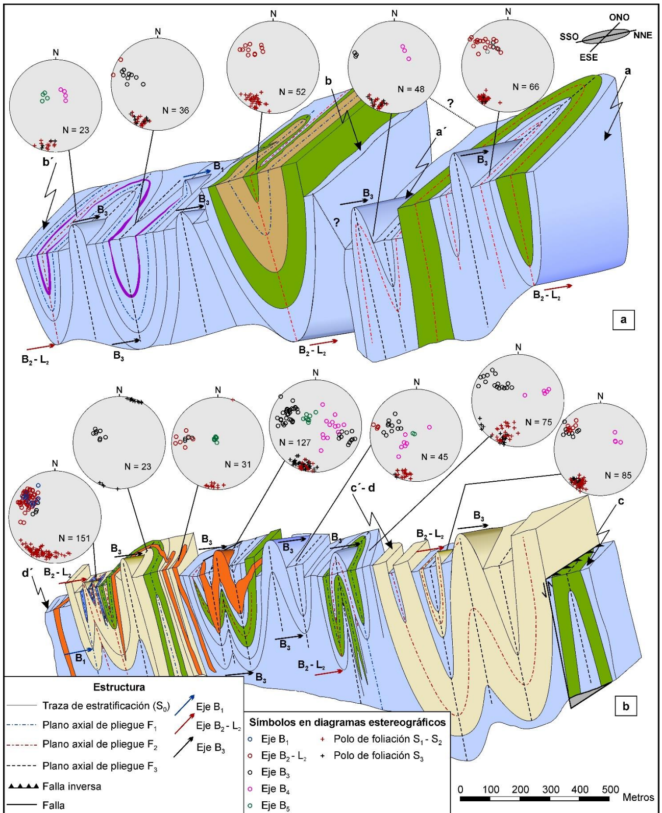
Figura 4.5. Blocks diagrama esquemático y proyección estereográfica de los elementos de fábrica de la Formación Nahuel Niyeu en las áreas al oeste (a) y norte (b) de Aguada Cecilio. Las referencias de las unidades geológicas se encuentran en la figura 4.1. Las estructuras D_3 de la Formación Nahuel Niyeu son equivalentes a las estructuras D_1 de los diques microgranodioríticos. Para ubicación ver las figuras 4.1 y 4.2. Los símbolos de las proyecciones estereográficas corresponden al rumbo e inclinación de ejes de pliegues (círculo) y a los polos de planos de foliación (cruces). N= número de datos. La proyección estereográfica es de igual área en hemisferio inferior.
