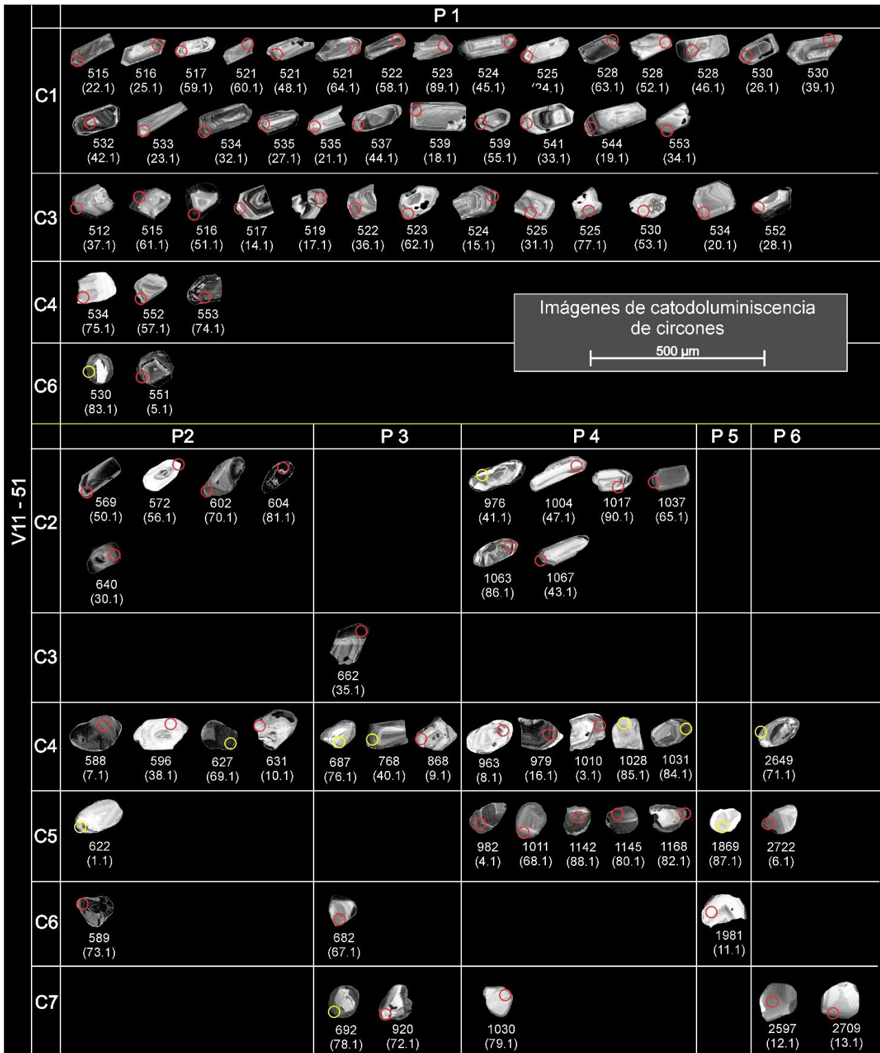
Figura 7.6. Imágenes de catodoluminiscencia de las poblaciones de circones de la muestra V11-51 agrupados de acuerdo a sus clases morfológicas (C1-C7). Cada spot analizado está indicado con un círculo (rojo, dato interpretado como de origen ígneo; amarillo, dato interpretado como de origen metamórfico). El origen ígneo o metamórfico fue interpretado teniendo en cuenta conjuntamente la estructura interna y la relación Th/U medida. El tamaño del spot es de 32 \mu m. Edad de las poblaciones de circones: población P1 (512-553 Ma), población P2 (569-640 Ma), población P3 (662-920 Ma), población P4 (963-1168 Ma), población P5 (1869-1981 Ma), población P6 (2597-2722 Ma). Edades U-Pb debajo de las imágenes. Para granos con edad \geq 1300 Ma se utilizó la edad ^{207}\text{Pb}/^{206}\text{Pb} , mientras que granos con edad \leq 1300 Ma se utilizó la edad ^{206}\text{Pb}/^{238}\text{U} . El número de spot está entre paréntesis. Sólo se muestran los circones correspondientes a los datos filtrados.
