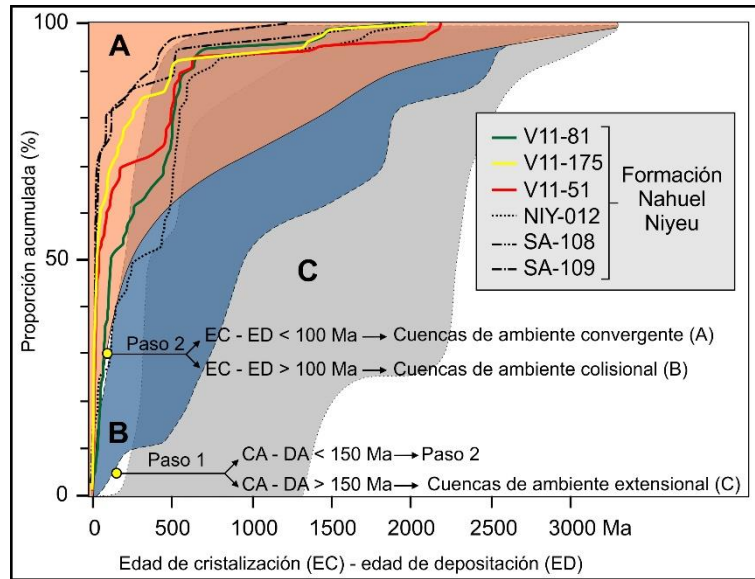
Figura 8.4. Proporción acumulada de la variación de la diferencia entre la edad de cristalización medida de un grano de circonio detrítico (EC) y la edad de deposición de la sucesión metasedimentaria de la Formación Nahuel Niyeu (ED). Este diagrama está basado en Cawood et al., 2012 . En este caso la edad de deposición está ajustada entre 516,6-515 Ma y 513,6 Ma (ver texto en la sección 8.1). Para simplificar se adoptó una edad de sedimentación de 515 Ma. Las zonas de color representan ambientes convergentes (A: naranja), colisionales (B: azul) y extensionales (C: gris). Las cuencas de ambientes extensionales tienen EC-ED mayores que 150 Ma en el 5% más joven de los circones (Paso 1). Las cuencas de ambientes convergentes tienen EC-ED menores que 100 Ma en el 30% más joven de los circones (Paso 2). Las cuencas asociadas a ambientes colisionales tienen EC-ED mayores que 100 Ma en el 30% más joven de los circones (Paso 2). Casi todas las muestras caen en el campo de las cuencas de ambiente convergente. Muestras V11-81, V11-170 y V11-51 (esta tesis), NIY-012 ( Pankhurst et al., 2006 ) y SA-108 y SA-109 ( Rapalini et al., 2013 ).
