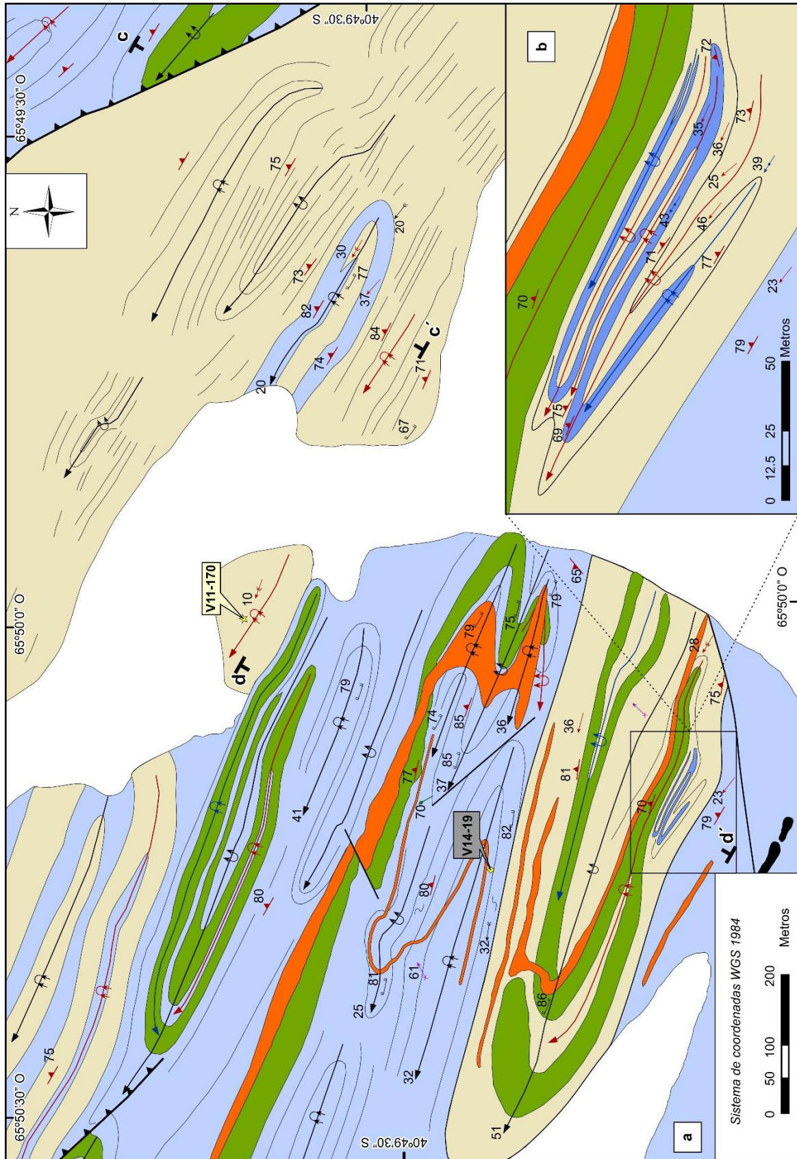
Figura 4.2. (a) Mapa geológico del área norte de Aguada Cecilio. El mapa incluye la ubicación de muestras y la traza del block diagrama c-c'-d-d' de la figura 4.5. (b) Detalle de los pliegues F 1 y F 2 en limbo de un pliegue F 3 . Las referencias del mapa se encuentran en la figura 4.1. Ubicación regional en la figura 1.1b.
