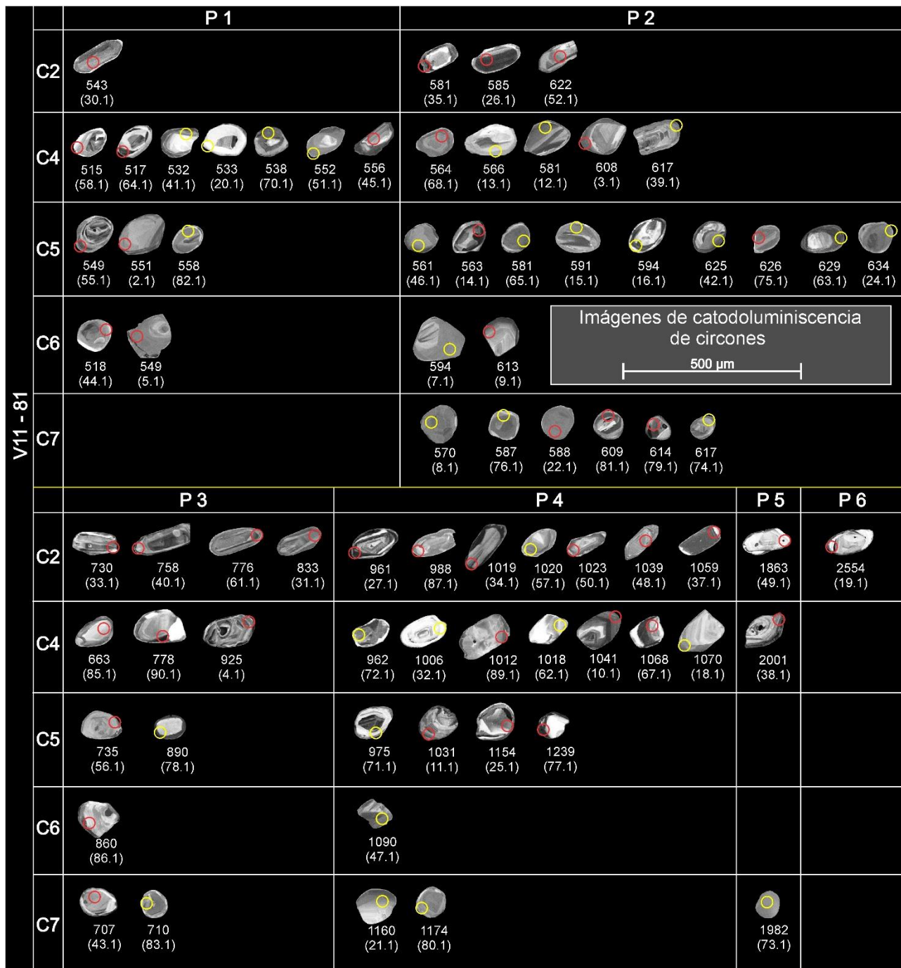
Figura 7.4. Imágenes de catodoluminiscencia de las poblaciones de circones de la muestra V11-81 agrupados de acuerdo a sus clases morfológicas (C2, C4, C5, C6 y C7). Cada spot analizado está indicado con un círculo (rojo, dato interpretado como de origen ígneo; amarillo, dato interpretado como de origen metamórfico). El origen ígneo o metamórfico fue interpretado teniendo en cuenta conjuntamente la estructura interna y la relación Th/U medida. El tamaño del spot es de 32 \mu m. Edad de las poblaciones de circones: población P1 (515-558 Ma), población P2 (561-634 Ma), población P3 (663-925 Ma), población P4 (961-1239 Ma), población P5 (1863-2001 Ma), población P6 (2554 Ma). Edades U-Pb debajo de cada imagen. Para granos con edad \geq 1300 Ma se utilizó la edad ^{207}\text{Pb}/^{206}\text{Pb} , mientras que para granos con edad \leq 1300 Ma se utilizó la edad ^{206}\text{Pb}/^{238}\text{U} . El número de spot está entre paréntesis. Sólo se muestran los circones correspondientes a los datos filtrados.
