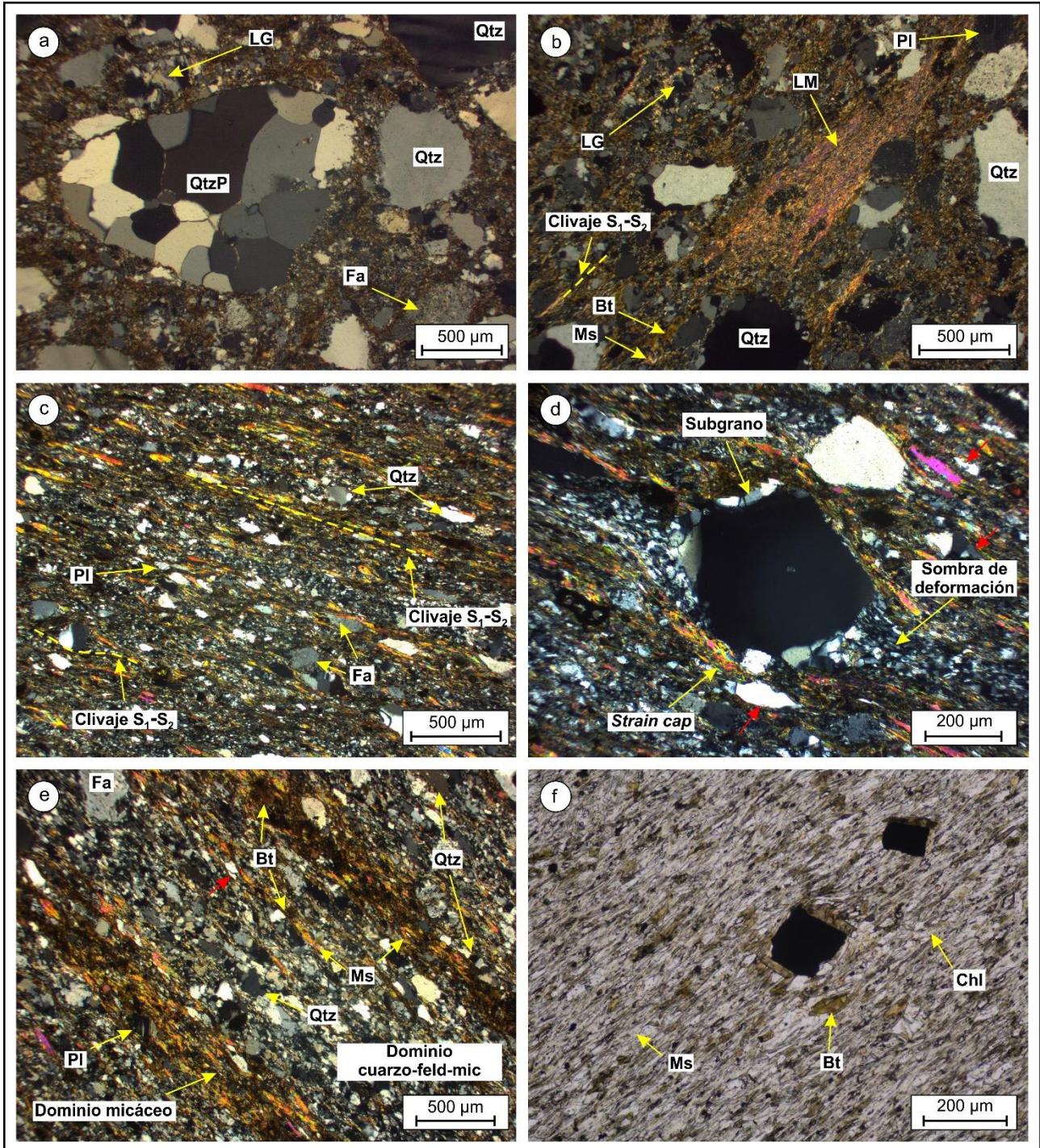
Figura 4.8. Fotomicrografías de las metasedimentitas de la litofacies verde grisácea en el área de Aguada Cecilio. (a), (b), (c), (d) y (e) Fotomicrografías tomadas con luz transmitida y nicols cruzados. (f) Fotomicrografía tomada con luz transmitida y nicols paralelos. Minerales metamórficos: Bt (biotita), Chl (clorita), Ep (epidoto), Ms (muscovita). Granos detríticos: Fa (feldespato alcalino), LG (líticos ígneos graníticos), LM (filita-pizarra), Pl (plagioclasa), Qtz (cuarzo), QtzP (cuarzo policristalino). (a) y (b) Metagrauwaca lítica masiva con granos detríticos, subredondeados y subangulosos, de cuarzo, feldespato alcalino, plagioclasa, y fragmentos líticos metamórficos (cuarzo policristalino y filita) e ígneos (microgranitos). El cuarzo policristalino muestra textura granoblástica. Los detritos están rodeados de una matriz recrystalizada que contiene una paragénesis metamórfica de biotita + muscovita + clorita + cuarzo + albita + clinozoisita + epidoto + turmalina. Notar las bandas de deformación y los subgranos y nuevos granos en los bordes de los detritos de cuarzo. El clivaje S_1-S_2 está pobremente desarrollado. Las fotomicrografías (a) y (b) corresponden a la muestra V11-81. (c) Metagrauwaca feldespática foliada con clivaje continuo S_1-S_2 . Cuarzo, feldespato alcalino y plagioclasa son granos detríticos relicíticos. Esta roca presenta una paragénesis mineral de biotita + muscovita + clorita + cuarzo + albita + epidoto + clinozoisita + turmalina. (d) Detalle de granos detríticos de cuarzo y feldespato alcalino de la sección delgada de la fotomicrografía (c). Estos granos se encuentran aplanados y estirados según el clivaje S_1-S_2 . El cuarzo del centro de la fotomicrografía muestra sombras de deformación ( strain shadow ), strain cap y subgranos en sus bordes. (e) Metagrauwaca feldespática laminada con dominios micáceos y cuarzo-feldespático-micáceos que definen un clivaje disyuntivo S_1-S_2 . La roca preserva granos detríticos muy deformados de cuarzo, plagioclasa y feldespato alcalino. Los dominios micáceos y la matriz recrystalizada de los ( continúa )
