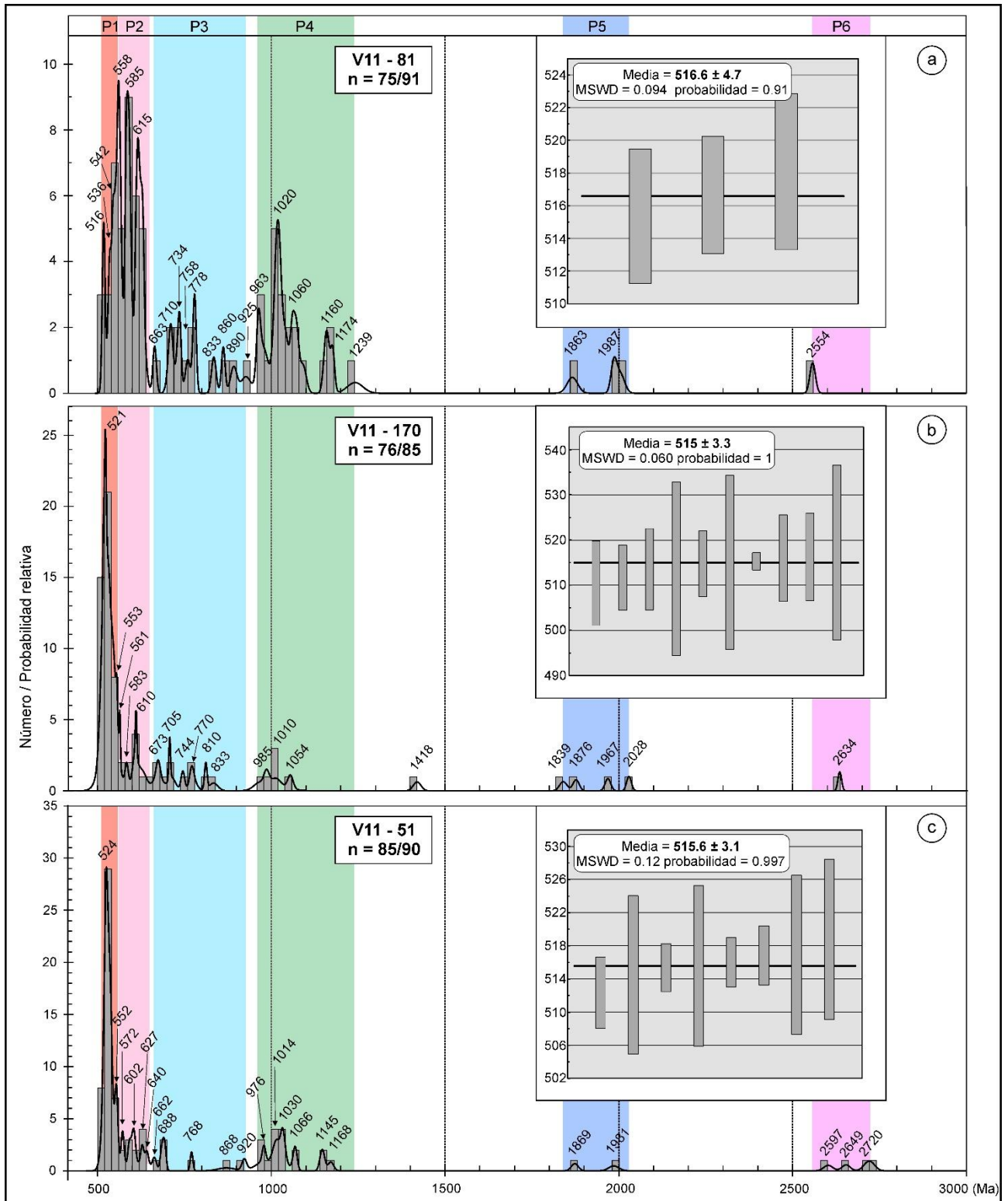
Figura 7.3. Diagramas de probabilidad relativa (curvas) y frecuencia (barras grises) de las edades de circones detríticos, y edad media ponderada de la población discreta más joven de granos de circon de las muestras V11-81 (a), V11-170 (b) y V11-51 (c). n = granos filtrados (con menos de 6% de ^{206}\text{Pb} de origen común y con menos de 10% de discordancia) / granos totales analizados. Los números encima de las curvas indican la edad del pico de probabilidad. Las barras de colores representan las edades de las poblaciones de los granos de circon. Todas las poblaciones discretas de circones más jóvenes tienen un origen ígneo. La incertidumbre para las medias ponderadas está dada en 2 sigmas. La altura de las barras de las medias ponderadas (edad de cada grano de la población más joven) está dada a 1 \sigma de error.
