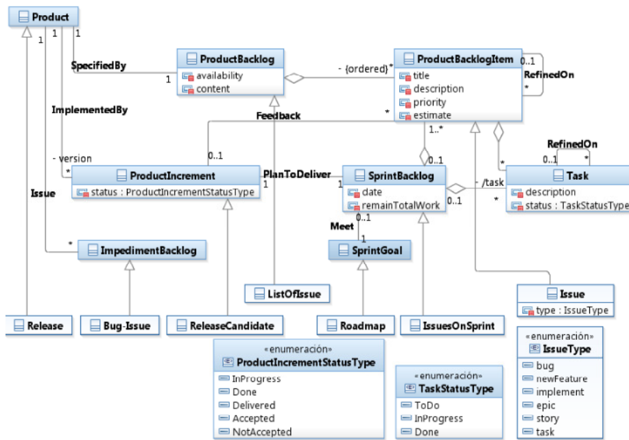
Fig. 8. Artefactos de Moodle en Scrum.
