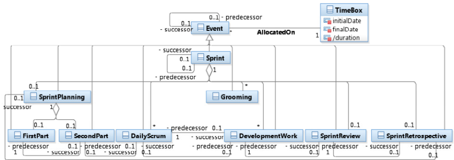
Fig. 4. Eventos definidos en Scrum.
