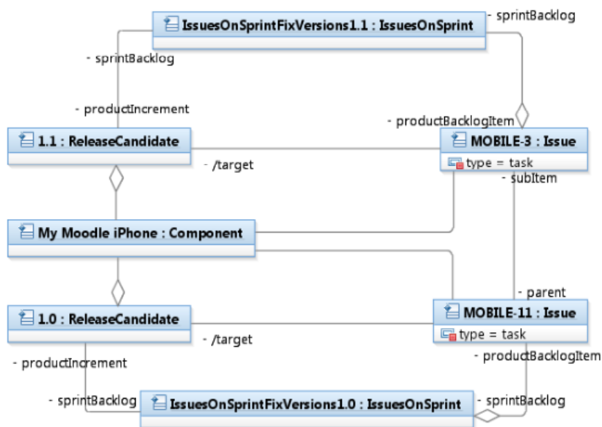
Fig. 10. Diagrama de objetos Issue MOBILE-3 y una sub-task, MOBILE11.
