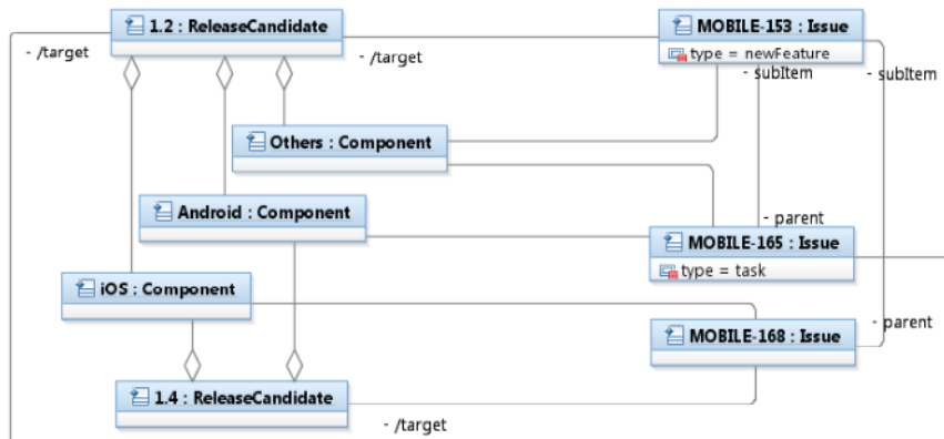
Fig. 12. Diagrama de objetos Issue MOBILE-153 (parcial).
