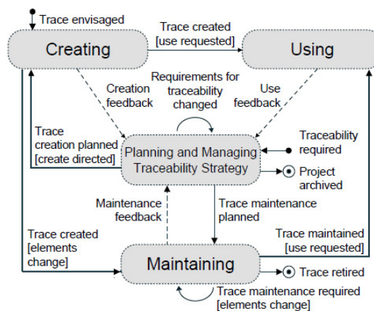
Fig. 2. Modelo del proceso de trazabilidad [17].
