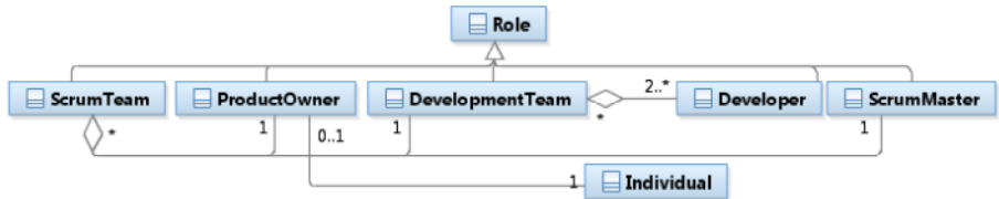
Fig. 3. Roles definidos en Scrum.
