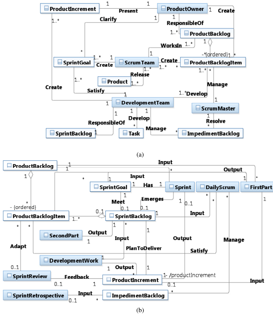
Fig. 6. Representación de Scrum. (a) Roles y artefactos. (b) Eventos y Artefactos
