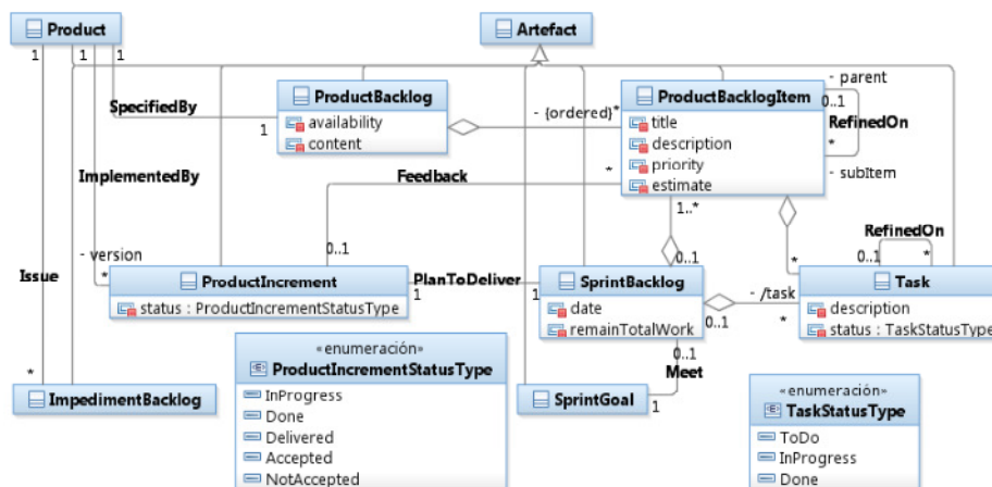
Fig. 5. Artefactos definidos en Scrum.
