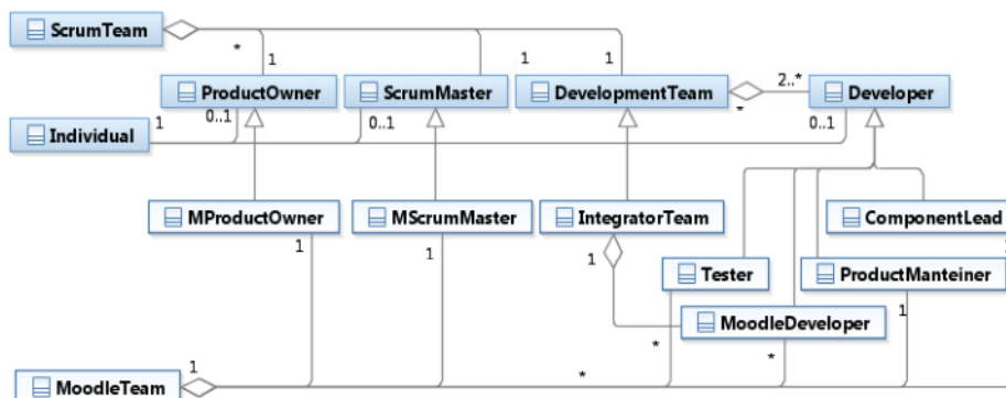
Fig. 7. Roles de Moodle en Scrum.
