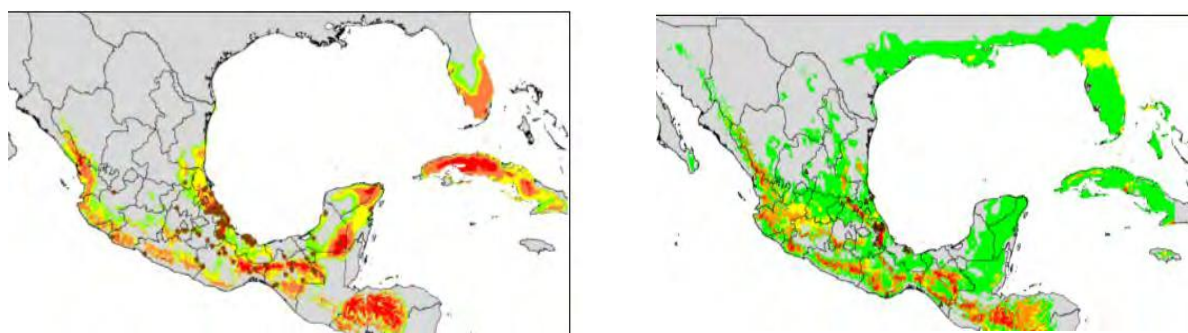
FIGURA 2. Probabilidad de ocurrencia de D. nigra (izquierda) y D. conzattii . (derecha). Colores más intensos representan mayor probabilidad.
