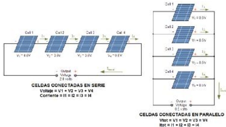
Figura 4 - Configuración de celdas fotovoltaicas en serie y paralelo
