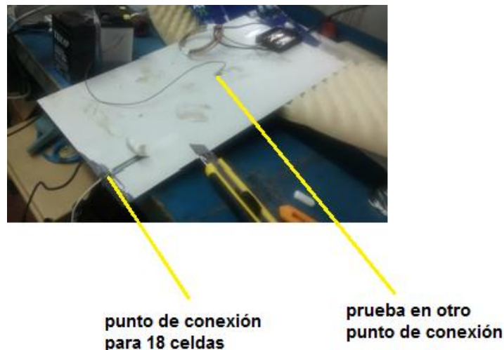
Figura 9 - Nuevos puntos de conexión del módulo
