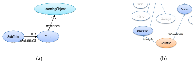
Fig. 5. Modificaciones a la ontología según directrices SNRD
