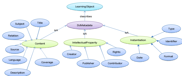
Fig. 4. Ontología DCOntoRep
