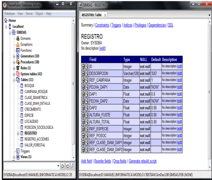
Fig. 2. Entorno FlameRobin
