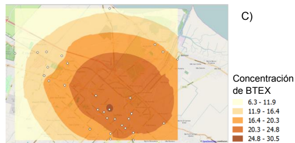
Fig 5. Interpolación por método de kriging ordinario para las concentraciones de benceno y BTEX en invierno 09 (A, B) y primavera 08 (C). Las concentraciones se encuentran expresadas en \mu\text{g}/\text{m}^3 . Los puntos blancos representan los puntos de muestreo.
