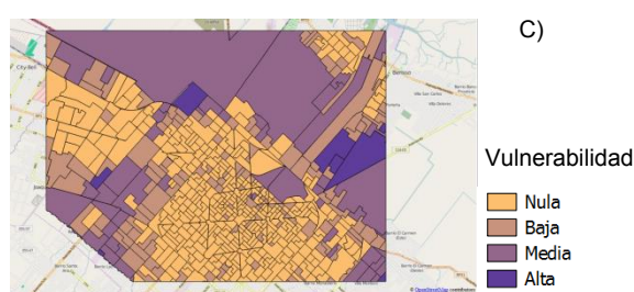
Fig. 6 Zona de riesgo de padecer cáncer clasificado según el grado de vulnerabilidad según los valores aceptables de: A) OMS para adultos en invierno 2009, B) EPA para niños en invierno 2009, C) EPA niños en primavera 2008.
