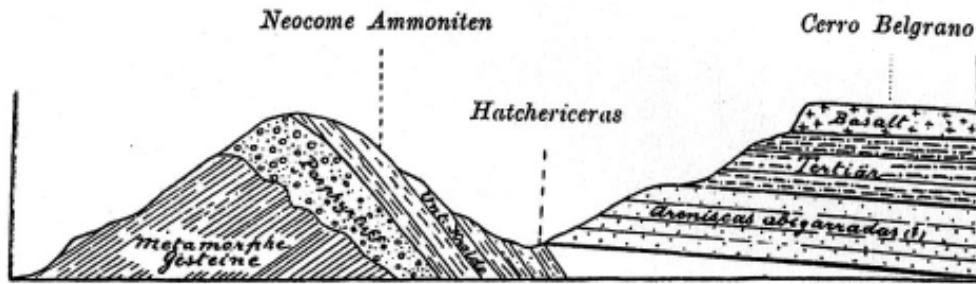
Figura 5. Estratigrafía de la zona norte del lago Belgrano, Santa Cruz (Hauthal, en Wilckens, 1905).
