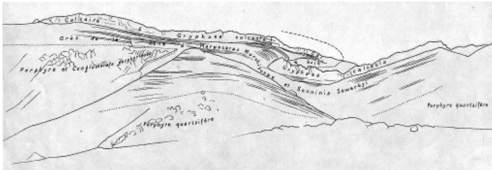
Figura 7. Esquema del Jurásico de Bardas Blancas, Mendoza, según Burckhardt (1900a).
