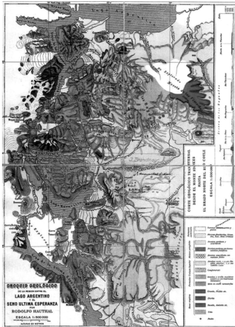
Figura 6. Mapa geológico de la región entre lago Argentino y el Seno de la Última Esperanza (Hauthal, en Wilckens, 1907a).
