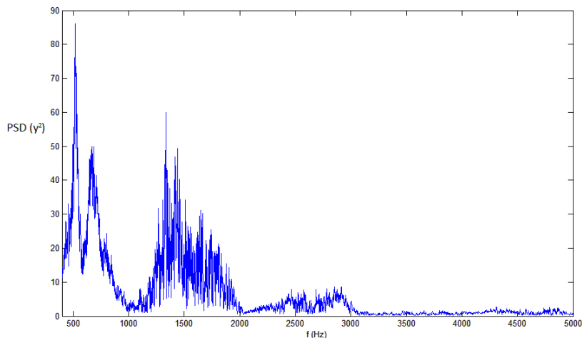
Figura 9: PSD sin el tubo (radial)
