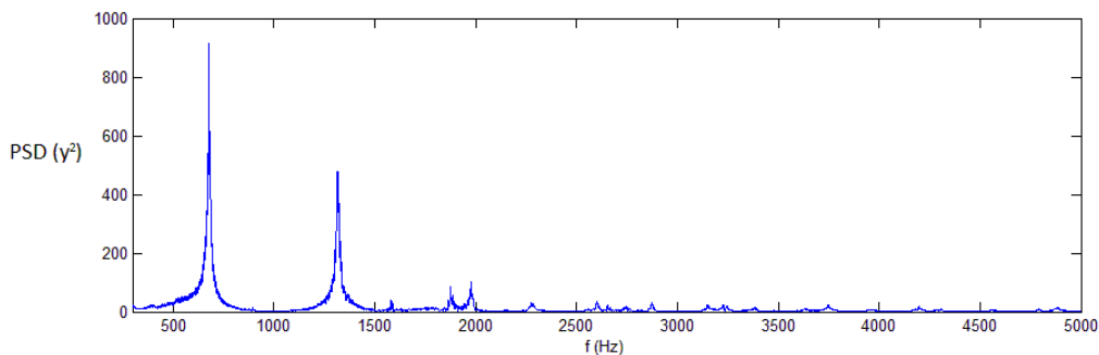
Figura 7: PSD con el tubo (longitudinal)
