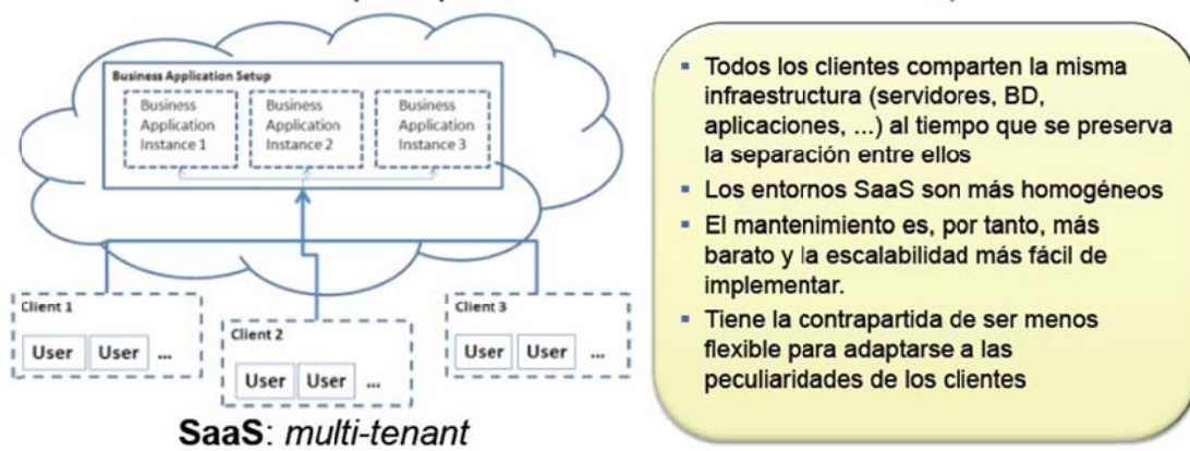
Fig. 62. SaaS multi-tenant
