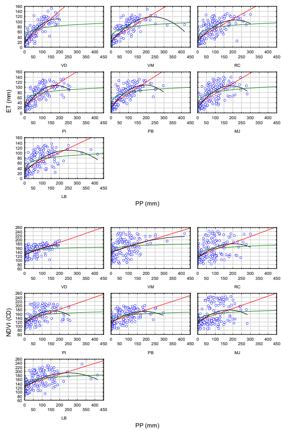
Fig. 2. Relación de los valores mensuales de precipitación (PP) con la evapotranspiración (ET) y NDVI (expresado en CD) en las estaciones meteorológicas de Córdoba.
