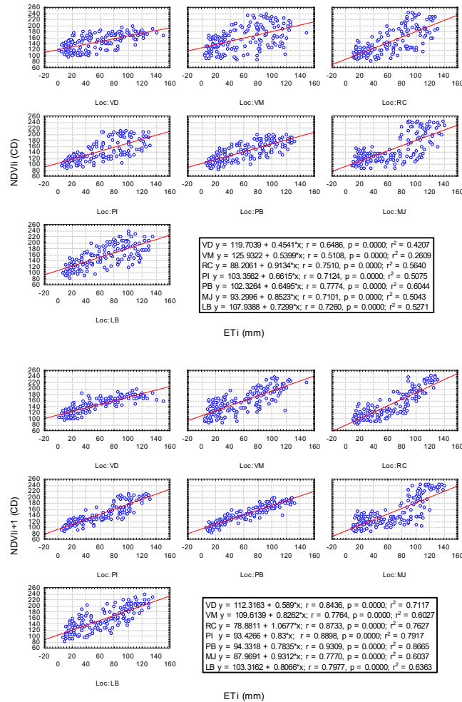
Fig. 3. Relación entre la evapotranspiración mensual (ET) y el NDVI en contadores digitales (CD) del mes actual i (arriba) y del mes posterior i+1 (abajo) en distintos sitios de Córdoba.
