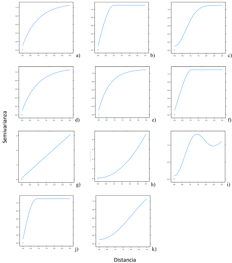
Fig. 2. Modelos de semivariogramas (semivarianza en función de distancia) disponibles en Fastmapping: a) exponencial, b) esférico, c) gaussiano, d) Matern, e) parametrización de Matern Stein, f) circular, g) lineal, h) power , i) wave , j) pentaesférico, k) hole .
