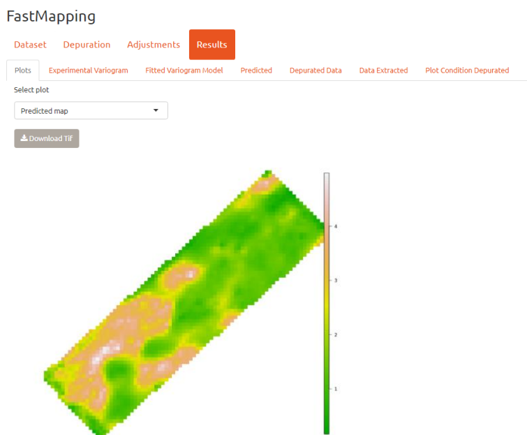
Fig. 5. Mapa de variabilidad espacial del rendimiento en un lote de soja
