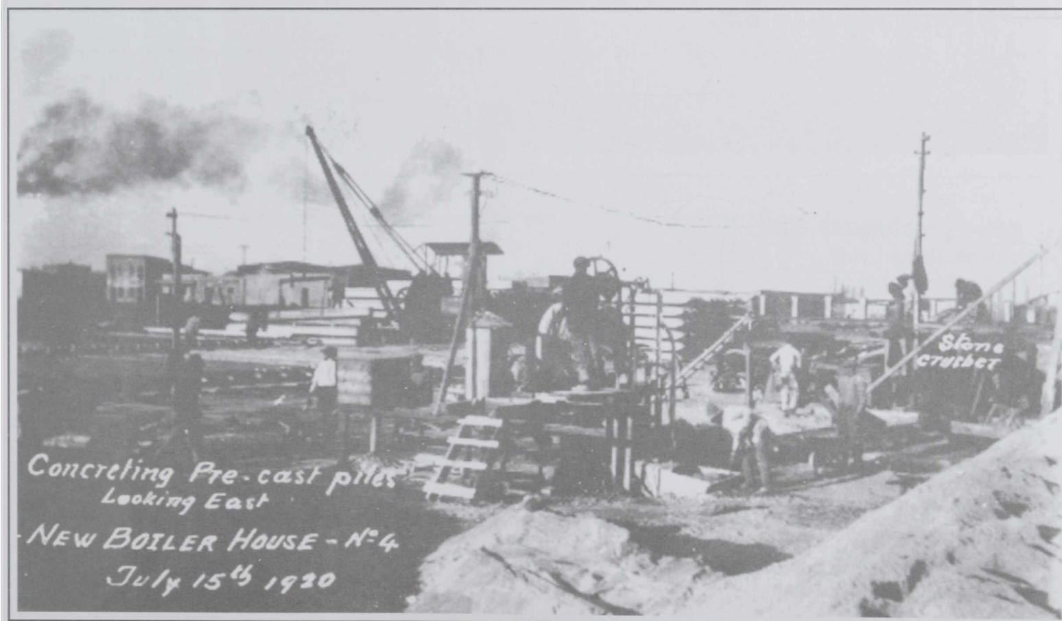
1920- Swift, construcción de pilotes en la zona nacional.
