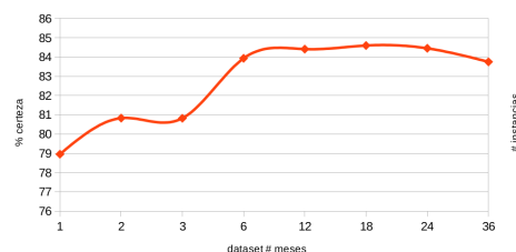
Figura 1. Análisis datasets
