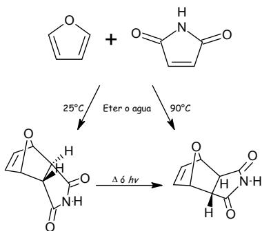
Figura 3. Fragmento de la ruta sintética desarrollada por Kwart y Burchuk[14]
