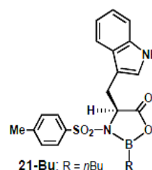
Figura 14. Catalizador 21-Bu [25]
