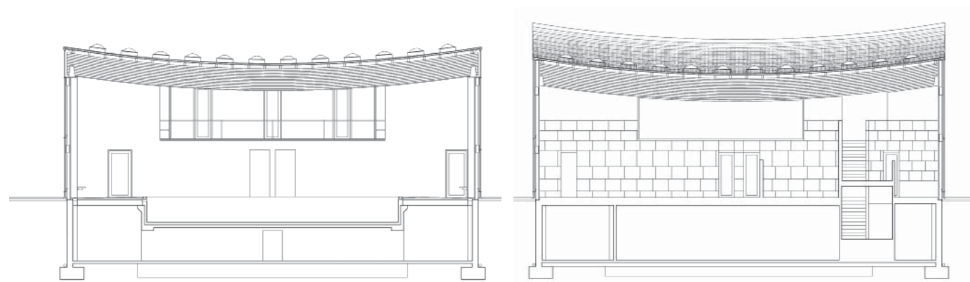
SECCIONES TRANSVERSALES
