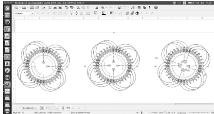
Fig. 10. Esquemas circulares de bobinados Bobinados de una fase con 1, 2 y 4 ramas en paralelo, respectivamente
