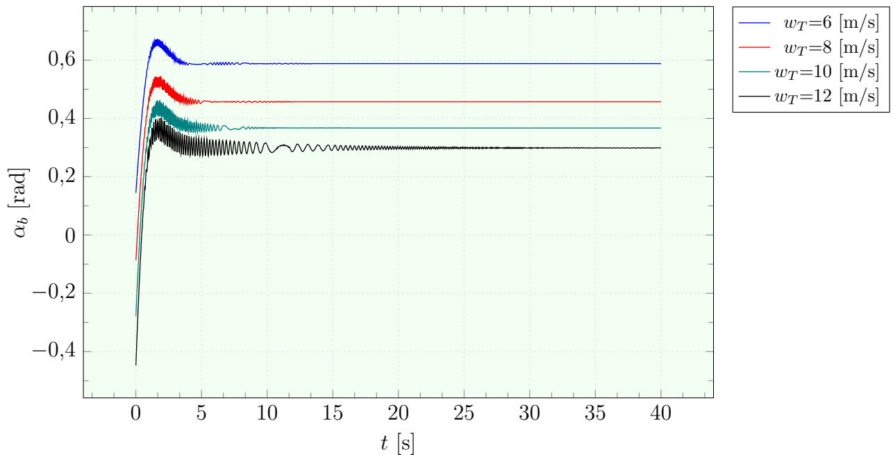
Figura 50: Ángulo de ataque de la pala b en el sistema equilibrado
