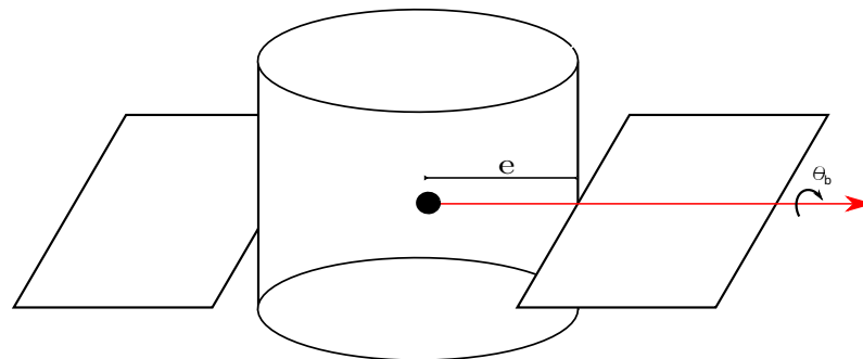
Figura 4: Esquema del pararrotor y definición del ángulo de paso.
