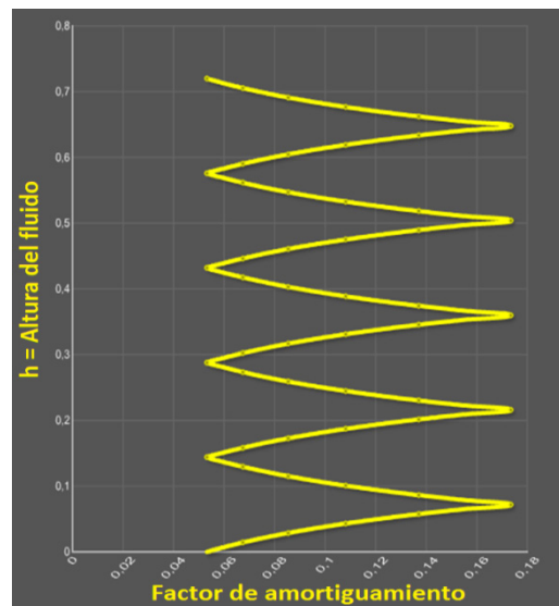
Figura 7. Variación del factor de amortiguamiento en función de la altura del fluido.
