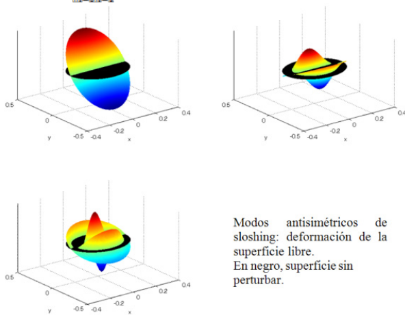
Figura 3. Modos antisimétricos de sloshing.
