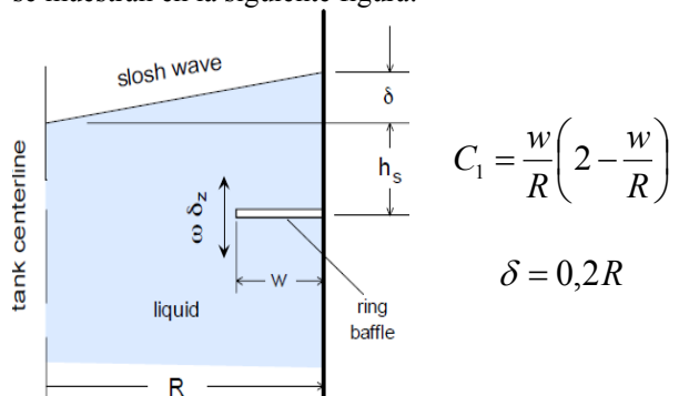
Figura 4 – Parámetros de la ecuación (2)
