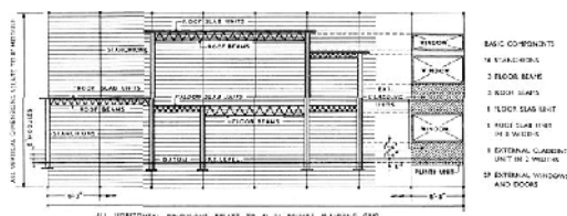
Fig. 22. Sistema de prefabricación Hills para edificios escolares, corte. Benevolo, L. (1974). Historia de la Arquitectura Moderna (2ª. ed.). Barcelona: Gili.
