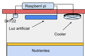
Figura 2. Diagrama de la cámara de germinación.
