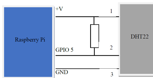
Figura 6. Conexiones del sensor DHT22 con el Puerto GPIO.
