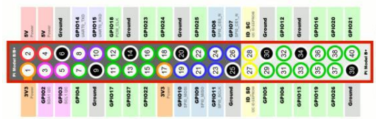
Figura 4. Salidas GPIO de Raspberry Pi.
