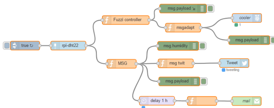
Figura 7. Diagrama de nodos del sistema de monitoreo de la cámara de germinación.
