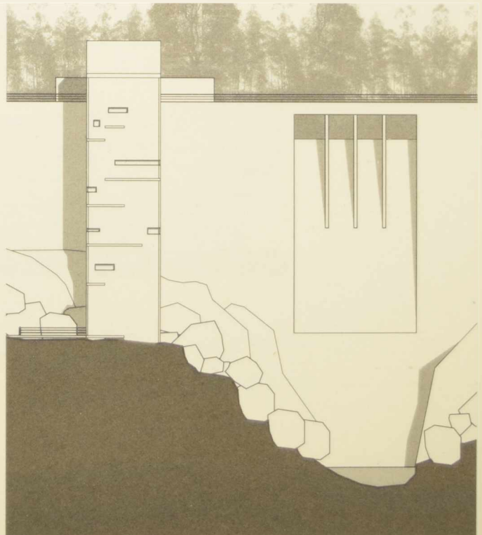
alzado elevation
