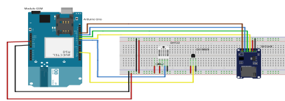
Fig. 1. Protótipo de monitoramento de temperatura do resfriador de leite.
