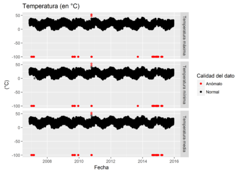
Figura 2. Exploración de outliers en la variable temperatura.
