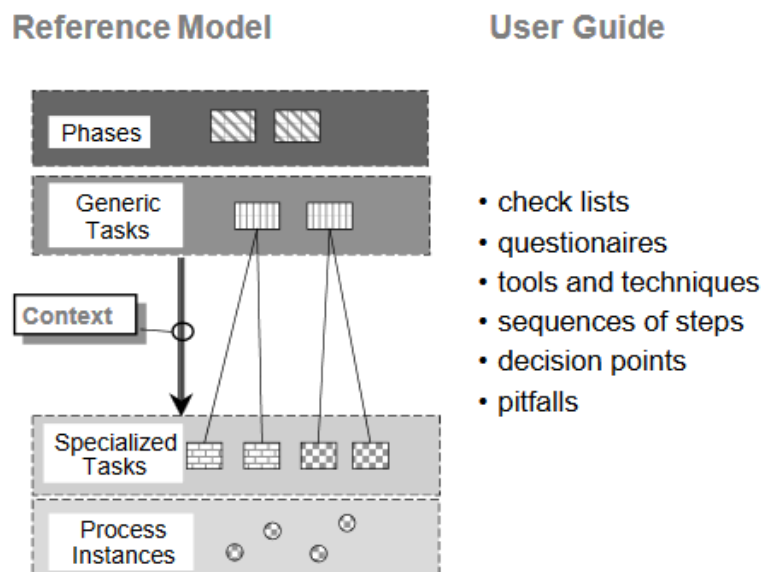
Figura 1. Fases de la metodología CRISP-DM [6].
