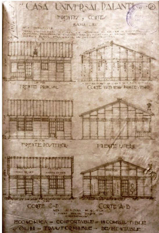
Figura 3: Casa Universal Palanti, Vistas y cortes de vivienda tipo realizada con el sistema Palanthome. 1923
