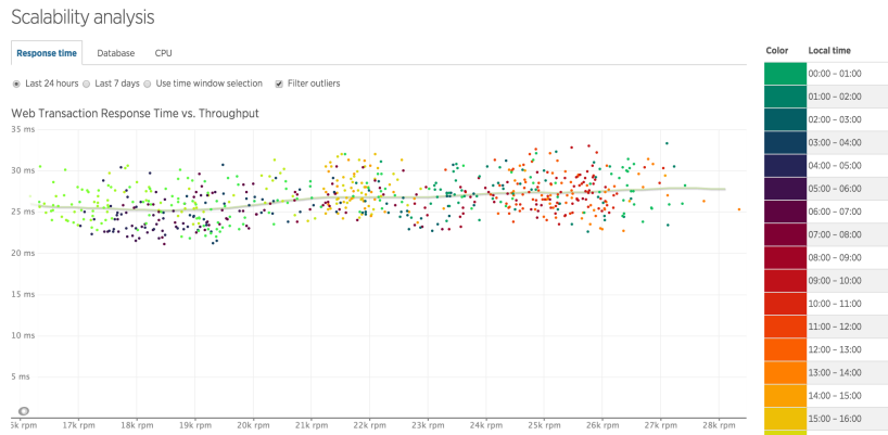
Figura 15: Análisis de escalabilidad de Lumen: tiempo de respuesta vs solicitudes por minuto. Fuente: darwinbiler.com [36]
