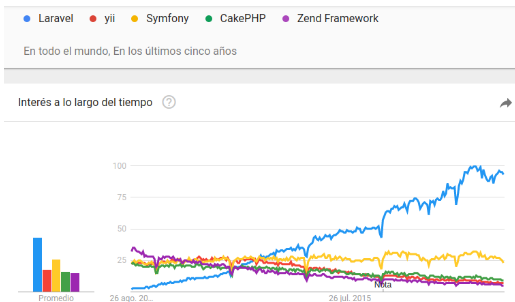
Figura 13: Tendencia en búsquedas sobre los principales Frameworks PHP en los últimos 5 años. Fuente: Google Trends[35]
