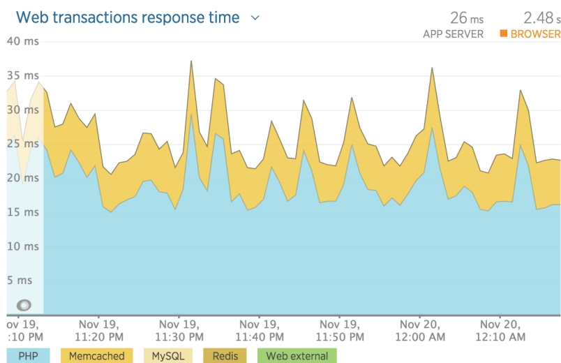
Figura 14: Tiempo de respuesta de las transacciones web con Lumen para aproximadamente 50k solicitudes por minuto. Fuente: darwinbiler.com [36]
