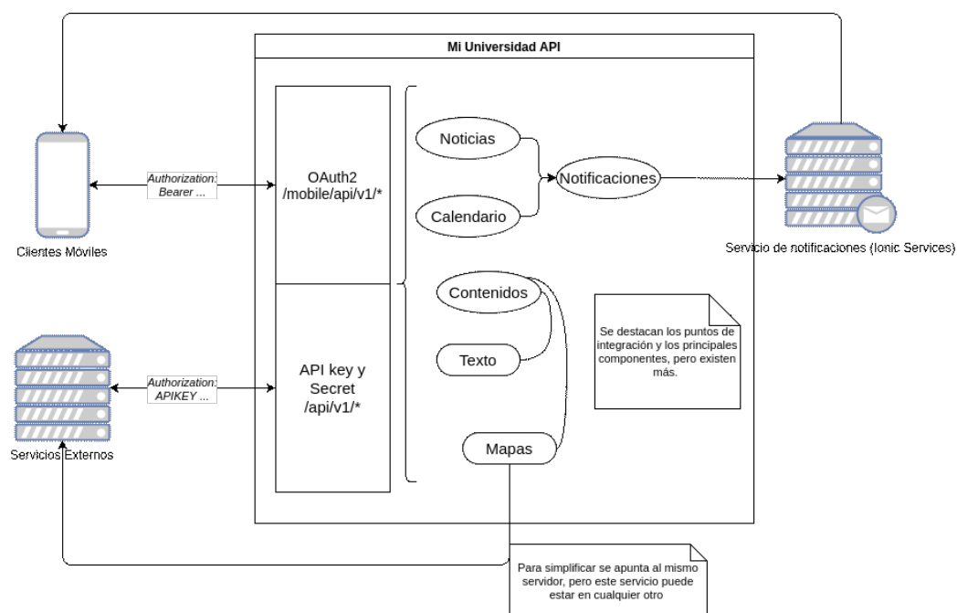
Figura 34: Diagrama de componentes de la API de Mi Universidad
