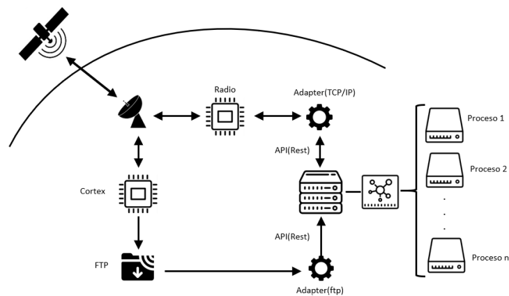
Figura 1. Arquitectura conceptual
