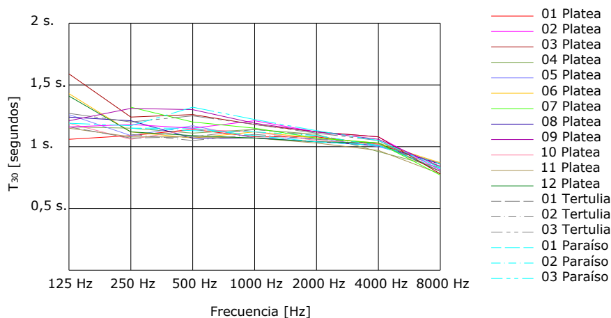
Figura 7. T_{30} [s] - Fuente lateral izquierdo escenario.
