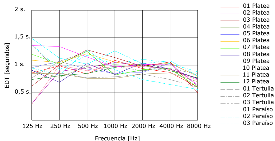
Figura 9. EDT [s] – Fuente lateral izquierdo escenario.
