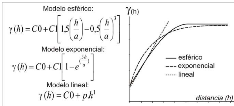
Figura 2: Ecuaciones de los modelos de variogramas empleados en los casos analizados. En todos se adicionaron dos estructuras: C0 (efecto pepita), C1 (contribución estructurada a la meseta), p (pendiente). A la derecha se esquematizan las curvas o recta generadas por cada ecuación.
