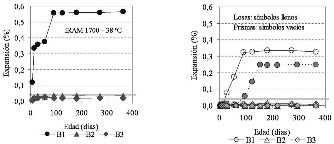
Figura 4. Serie B. Evolución de las expansiones. a) Izq. Ensayos normalizados. b) Der: medidas sobre losas y prismas ubicados junto a ellas.
