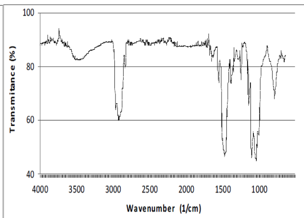
Figura 4- Madera modificada con la mezcla de ambos alcóidos
