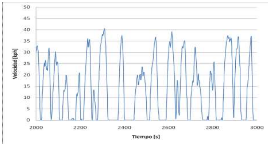
Gráfico N° 1: Ciclo de manejo
