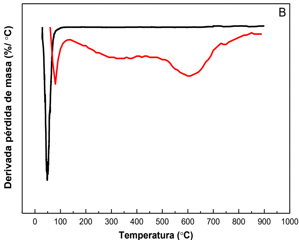
Figura 68. Análisis termogravimétrico de MCM-41 (negro) y MCM-41-NH 2 -CH 3 (rojo). (A) Análisis TGA y (B) 1 o Derivada.
