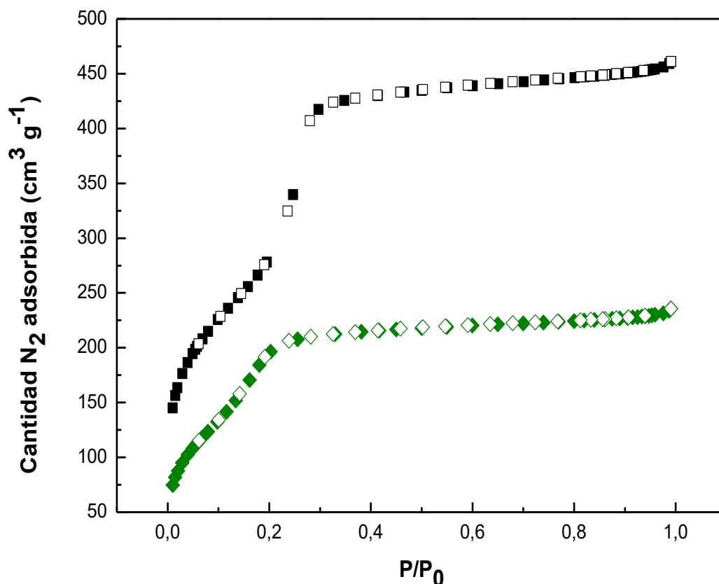
Figura 63. Isotherma de Adsorción-Desorción de N 2 para MCM-41 (cuadrados negros) y MCM-41-NH 2 -CH 3 (rombos verdes).
