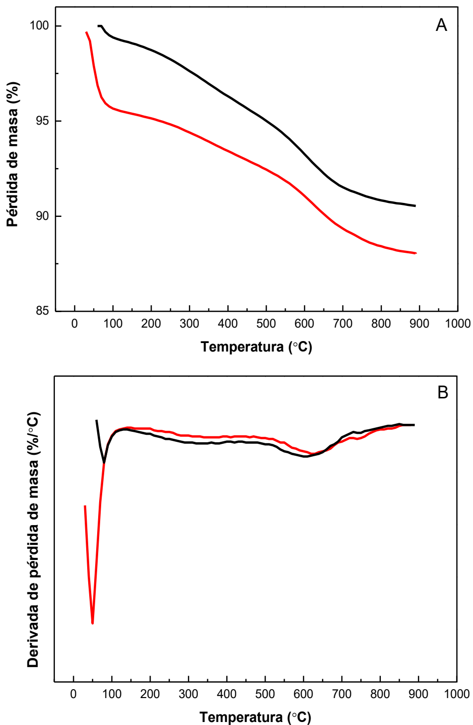
Figura 79. A) Análisis termogravimétrico de MCM-41-NH 2 -CH 3 (negra) y MCM-41-NH 2 -CH 3 -8h-pH 10 (rojo). B) 1 o Derivada.
