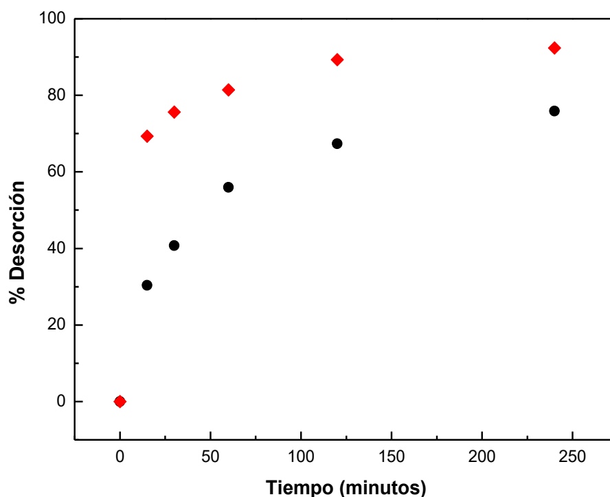
Figura 48. Desorción de Cr(VI): círculos (negros) pH= 8.0 ± 0.2 y rombos (rojos) pH= 10.0 ± 0.2 (Sc. NaOH).
