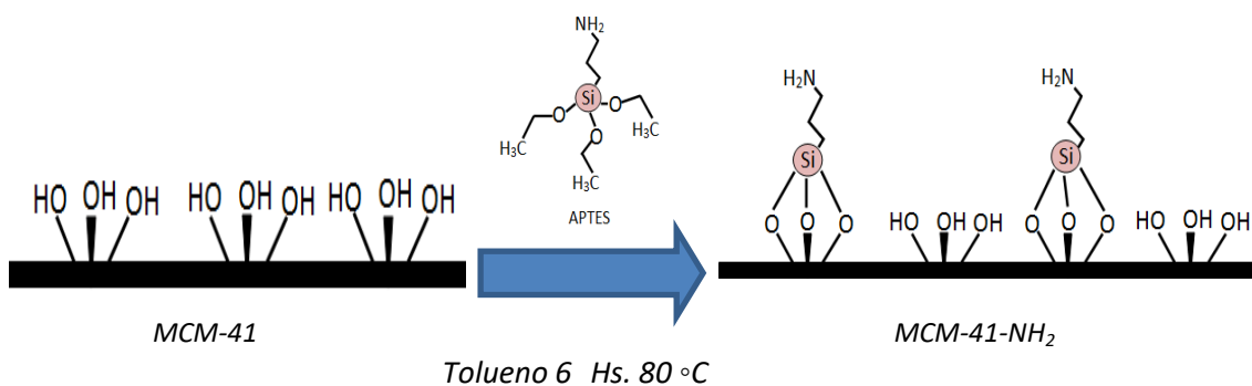
Figura 10. Esquema del proceso de funcionalización del sistema MCM-41-NH 2 .
