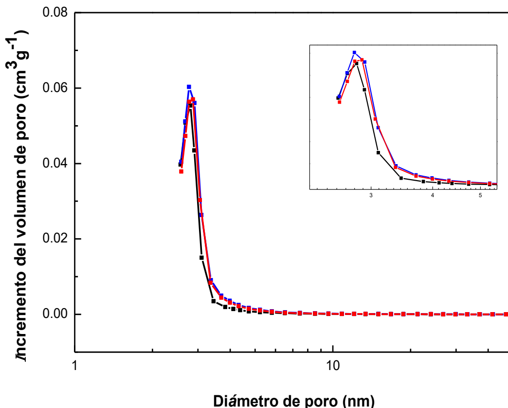
Figura 75. Distribución de diámetro de poro de MCM-41-NH 2 -CH 3 (negro), MCM-41-NH 2 -CH 3 - 1h-pH 10 (azul) y MCM-41-NH 2 -CH 3 -8h-pH 10 (roja) calculados empleando el modelo de BJH-KJS. El inserto corresponde a una ampliación de la zona 2 - 5 nm.
