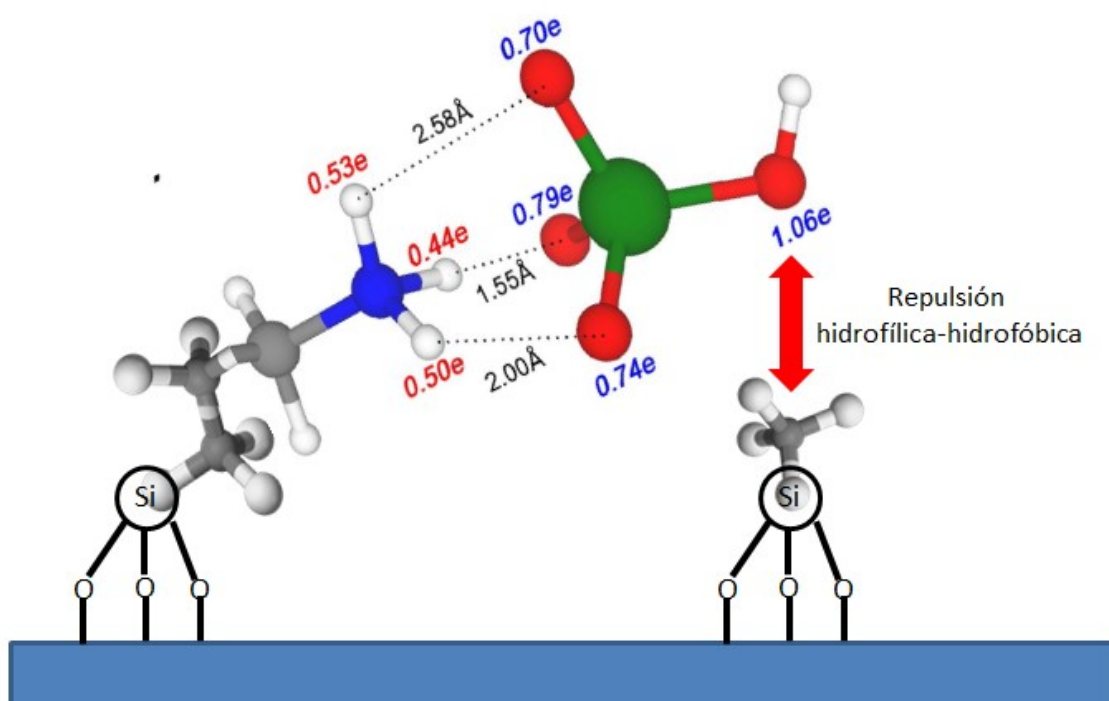
Figura 70. Esquema de la repulsión hidrofílica-hidrofóbica entre el HCrO 4 - y el grupo -CH 3 .
