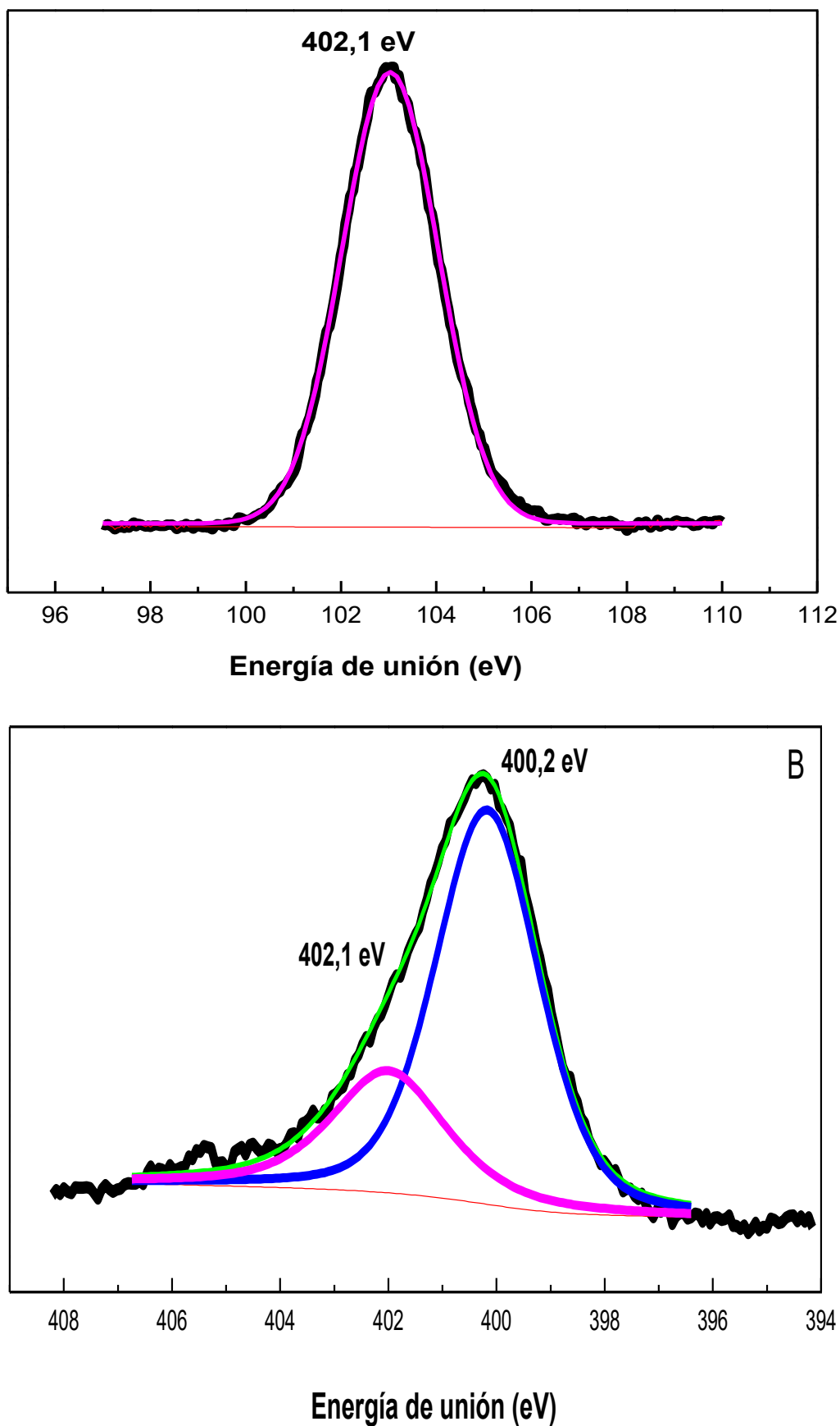
Figura 21. Espectros XPS de MCM-41-NH 2 A) en la región Si2p y B) la región N1s.
