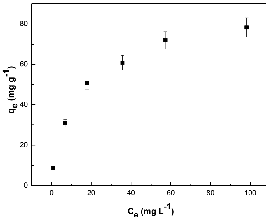
Figura 43. Isoterma de adsorción de Zn (II) por MCM-41.
