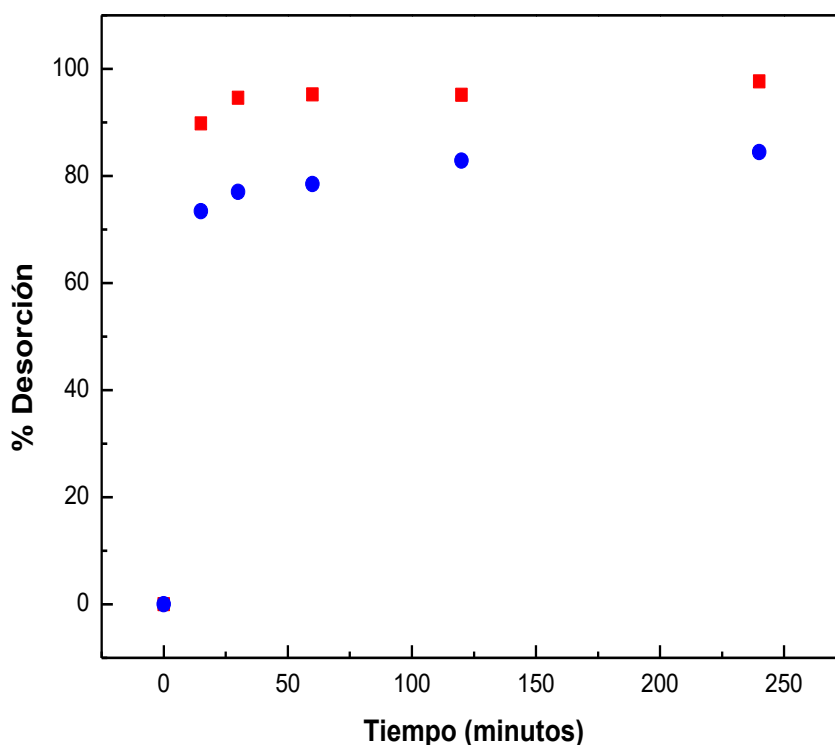
Figura 47. Desorción de Zn(II): círculos (azules) pH= 2.0 ± 0.2 y cuadrados (rojos) pH= 1.5 ± 0.2 (Sc. HCl).
