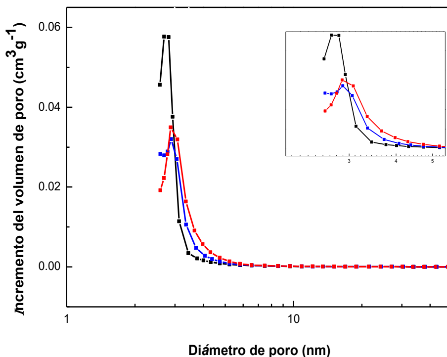
Figura 54. Distribución de diámetro de poro de MCM-41-NH 2 (negro), MCM-41-NH 2 -1h-pH 10 (azul) y MCM-41-NH 2 -8h-pH 10 (roja) calculados empleando el modelo de BJH-KJS. El inserto corresponde a una ampliación de la zona 2 - 5 nm.
