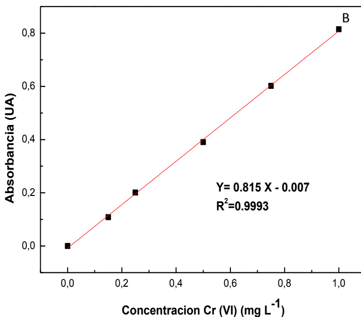
Figura 23 A). Espectro de absorción del complejo difenilcarbazona-Cr(III). B) Ejemplo de curva de calibración empleada en este trabajo de tesis.
