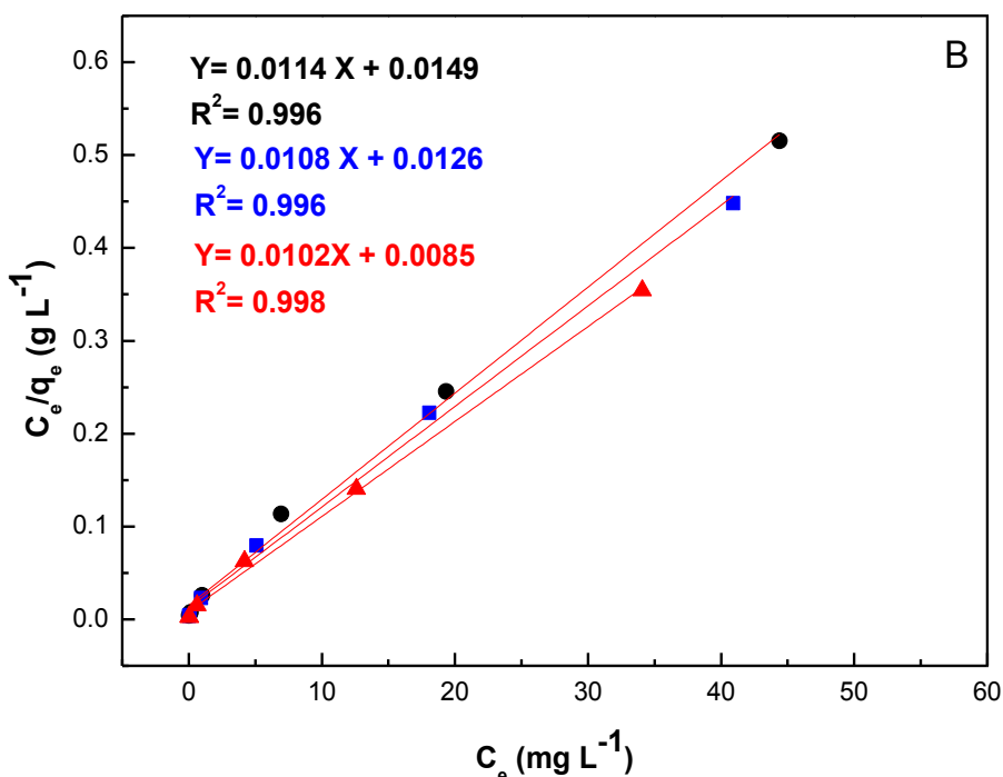
Figura 37. A) Isoterma de adsorción de Cr(VI) utilizando MCM-41-NH 2 a 25°C (círculos negros), 35°C (cuadrados azules) y 45°C (triángulos rojos). B) Ajuste realizado aplicando el modelo de Isoterma de Langmuir.
