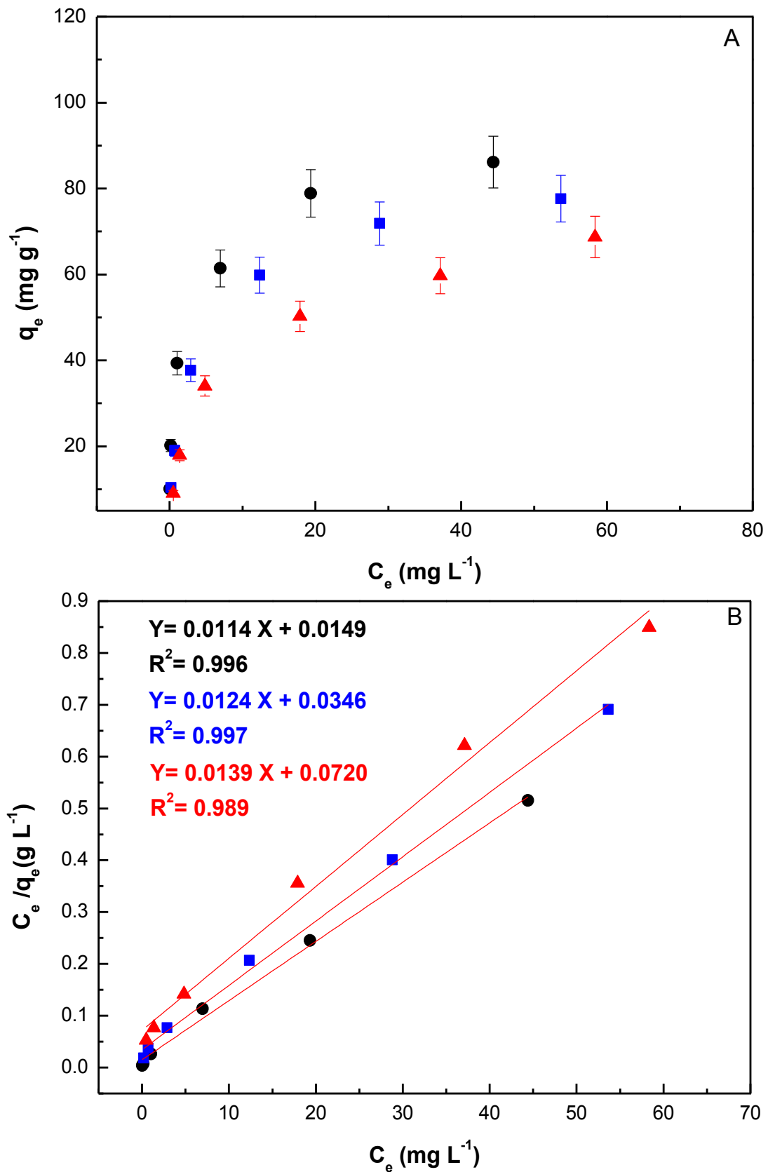
Figura 38. A) Isothermas de adsorción de Cr(VI) por MCM-41-NH 2 realizadas a 25°C y pH 2.2 a diferentes concentraciones de KCl: 0M (círculos negros), 0.01M (cuadrados azules) y 0.1M (triángulos rojos). B) Ajuste realizado aplicando el modelo de Isotherma de Langmuir.
