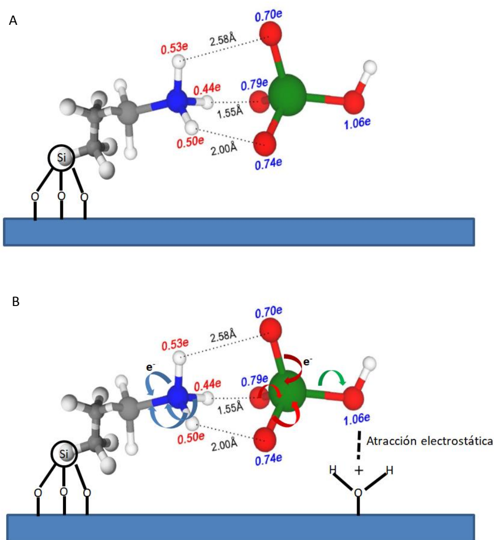
Figura 35. A- Interacciones entre las especies \text{-NH}_3^+ y \text{HCrO}_4^- y B- Interacción del \text{HCrO}_4^- adsorbido con los silanoles protonados ( \text{-Si-OH}_2^+ ). Las esferas blancas representan átomos de hidrógeno, mientras que las esferas grises, azules, rojas y verdes representan átomos de carbono, nitrógeno, oxígeno y cromo respectivamente. La cantidad de carga positiva (o negativa) de cada átomo está indicada por números en letras rojas (o azules).
