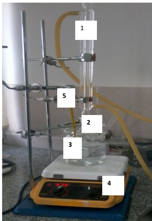
Figura 9. Sistema de funcionalización: 1-Conexión refrigerante; 2-Balón donde se coloca la muestra, el solvente y el APTES; 3-Baño de agua caliente para mantener constante la temperatura; 4-Plancha calefactora con control de agitación y temperatura; 5-termómetro.
