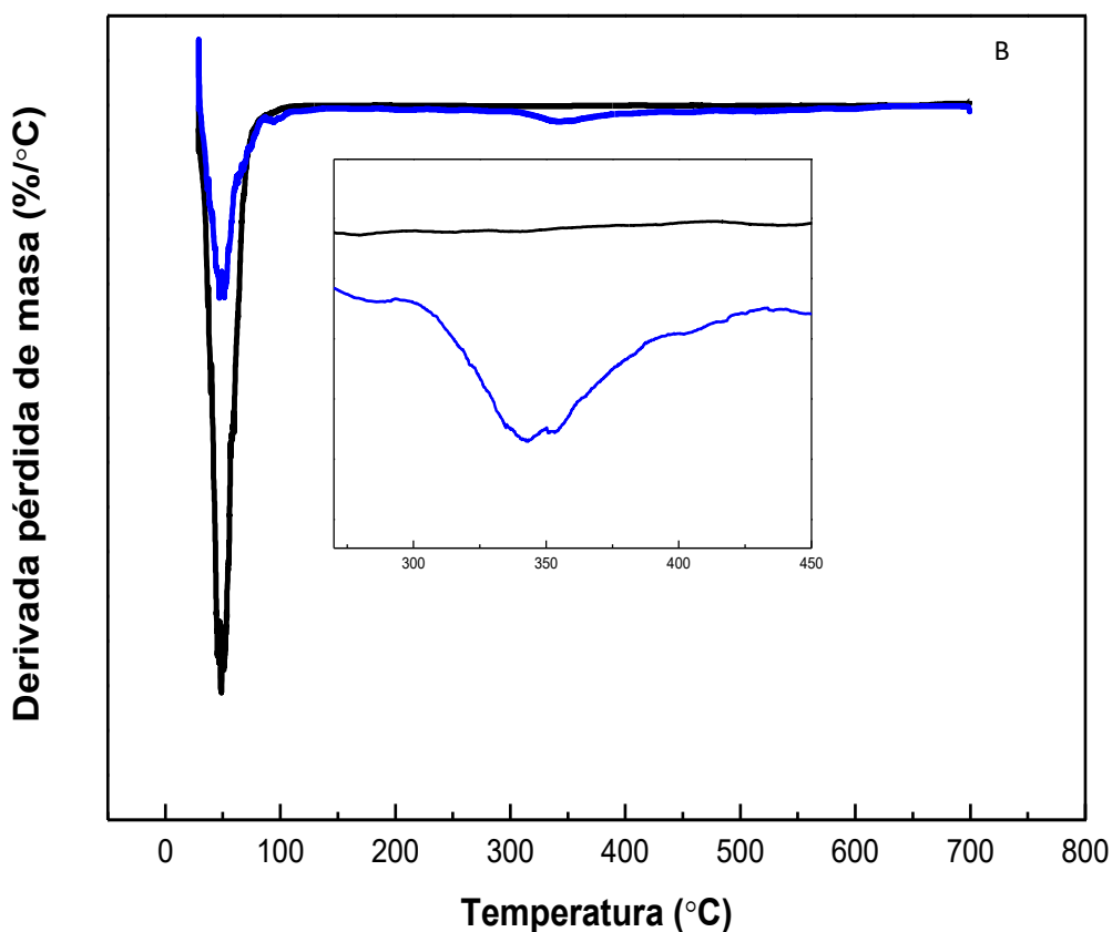
Figura 19. Análisis termogravimétrico de MCM-41 (negro) y MCM-41-NH 2 (azul). (A) Análisis TGA y (B) 1 o Derivada. Inserto, ampliación de la zona 250-450 °C.
