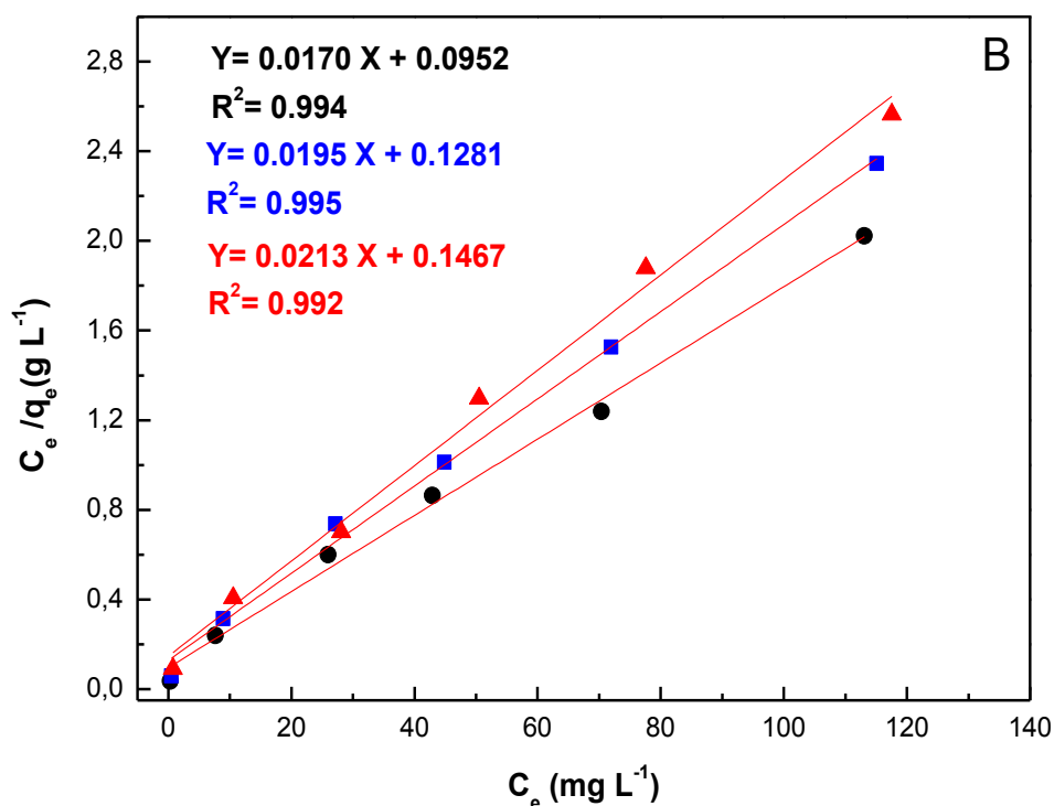
Figura 45. A) Isoterma de adsorción de Zn(II) por MCM-41-NH 2 realizadas a 25 °C y pH= 7.0 ± 0.2 a diferentes concentraciones de KCl: 0 M (círculo), 0.01 M (cuadrado) y 0.1 M (triángulo). B) Ajuste realizado aplicando el modelo de Isoterma de Langmuir.
