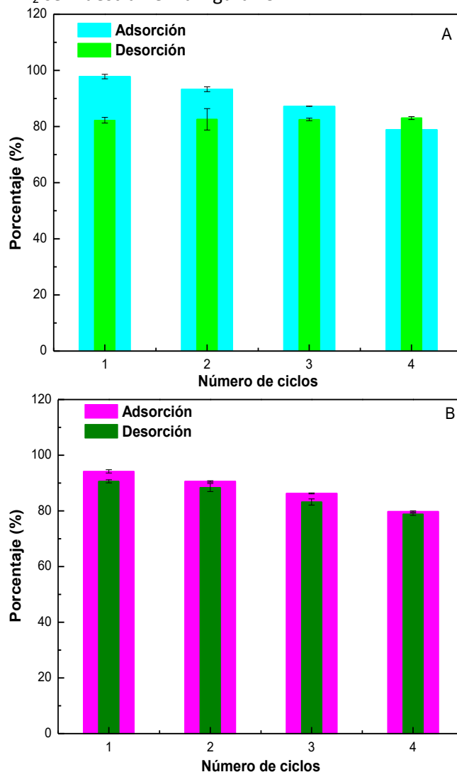
Figura 49. Ciclos de adsorción-desorción utilizando MCM-41-NH 2 para Cr(VI) (A) y para Zn(II) (B).
