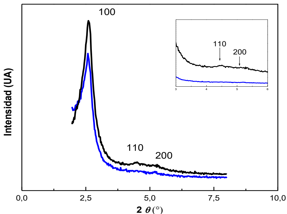
Figura 11. Patrones de difracción de rayos X a bajos ángulos. MCM-41 (negro) y MCM-41-NH 2 (azul). El inserto corresponde a una ampliación de la zona de 2\theta entre 3° y 6°.
