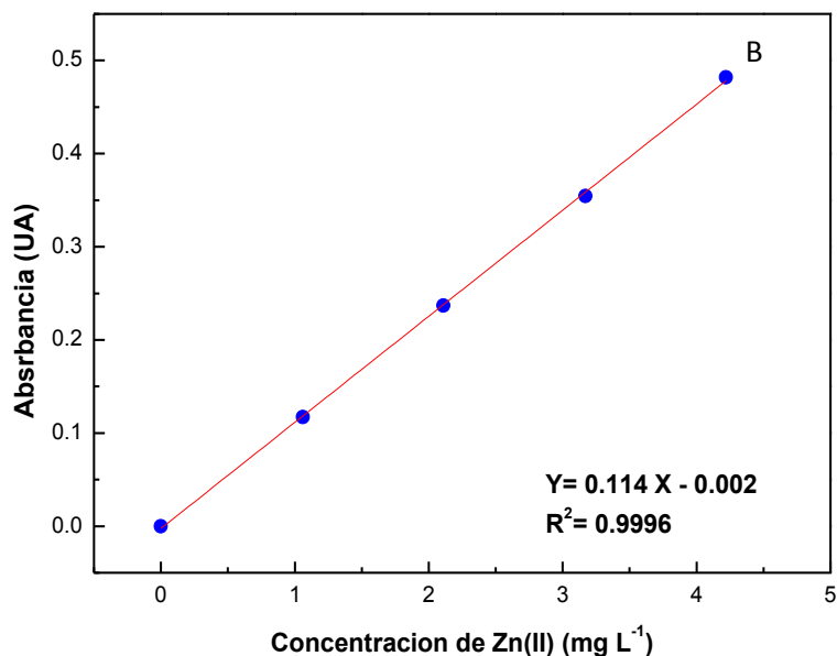
Figura 25 A). Espectro de absorción del complejo ditizona-Zn(II). B) Ejemplo de curva de calibración empleada en este trabajo de Tesis.
