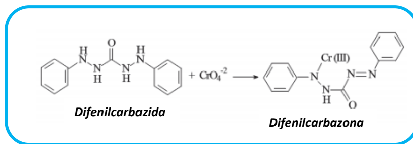
Figura 22. Estructura del complejo entre cromo hexavalente y 1,5 difenilcarbazida.
