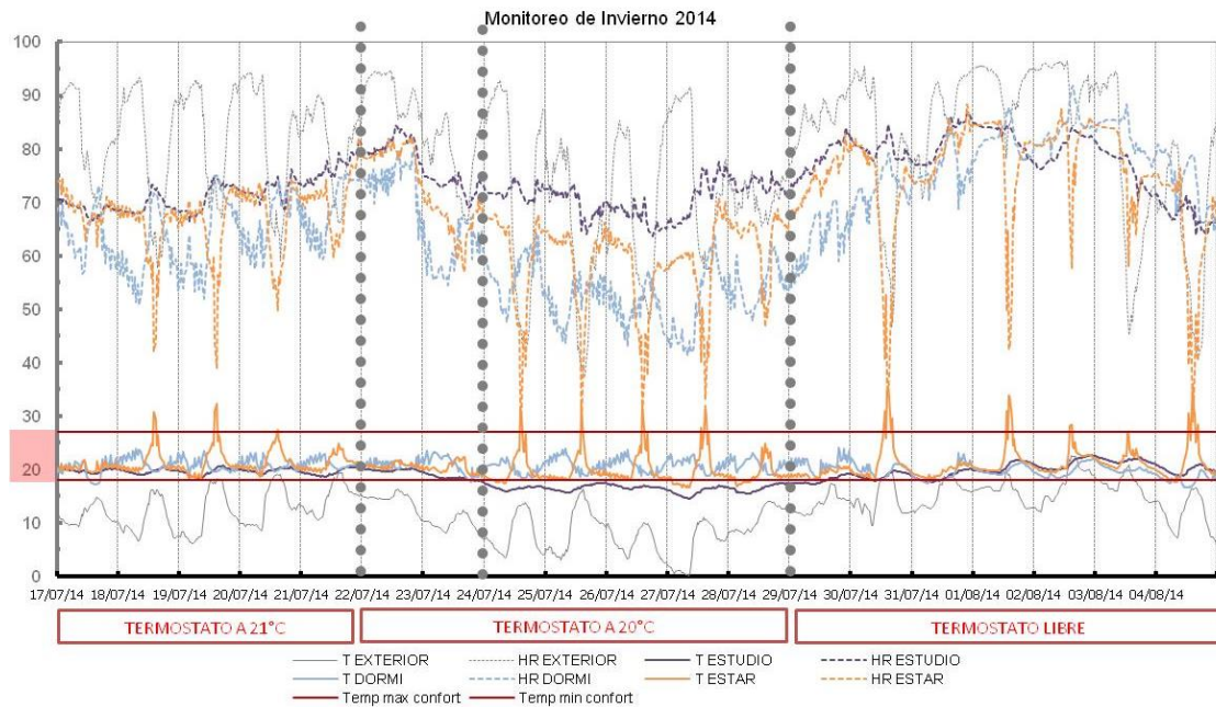
Figura 10 - Monitoreo higtotérmico invernla
