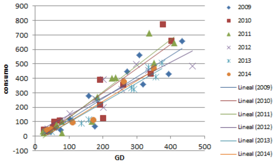
Figura 12 - Consumo mensual de gas respecto de grados día con base 20°C (GD 20 ) monitoreados
