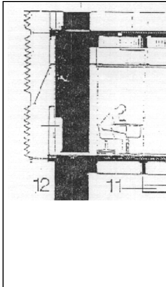
Figura 1 Detalle que muestra la resolución de los parasoles exteriores en las torres CAGLP. (1971)
