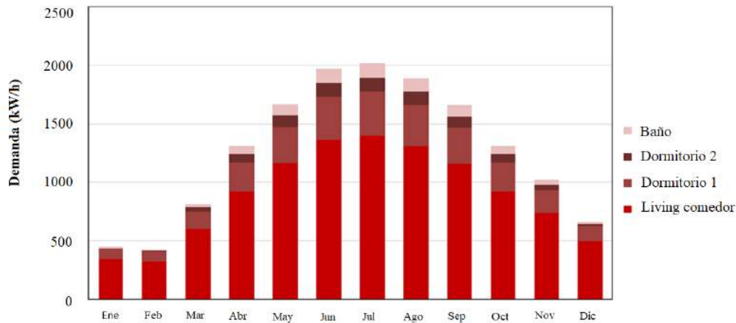
Figura 5. Distribución de demanda energética por local en estado base. Fuente: Elaboración de los autores.
