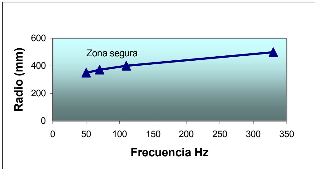
Figura N°11: Radio de curvatura admisible versus frecuencia de resonancia para celdas solares
