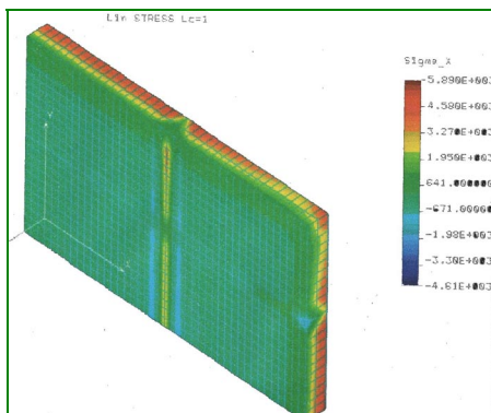
Figura N° 2: Análisis de una celda solar por el Método de Elementos Finitos
