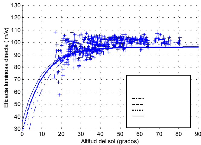
Figura 1. Variaciones de la eficacia luminosa directa con la altitud del sol y resultados modelo de Perez
