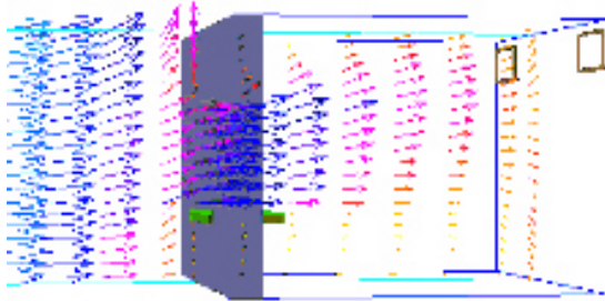
Fig 7 Simulación en computadora. Egreso de aire por dos aberturas
