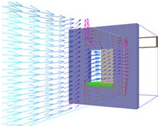
Fig 11 Simulación en Computadora. Abertura existente
