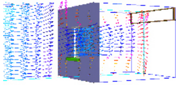
Fig 8 Simulación en computadora. Egreso de aire por una abertura longitudinal
