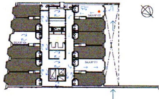
Fig 4 Ensayo en Túnel de Viento en Planta existente
