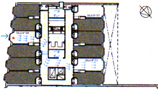
Fig 3 Ensayo en Túnel de Viento en Planta existente
