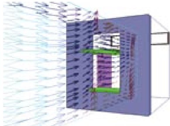
Fig 12 Simulación en Computadora. Prototipo de ventana pivotante con direcciones variables
