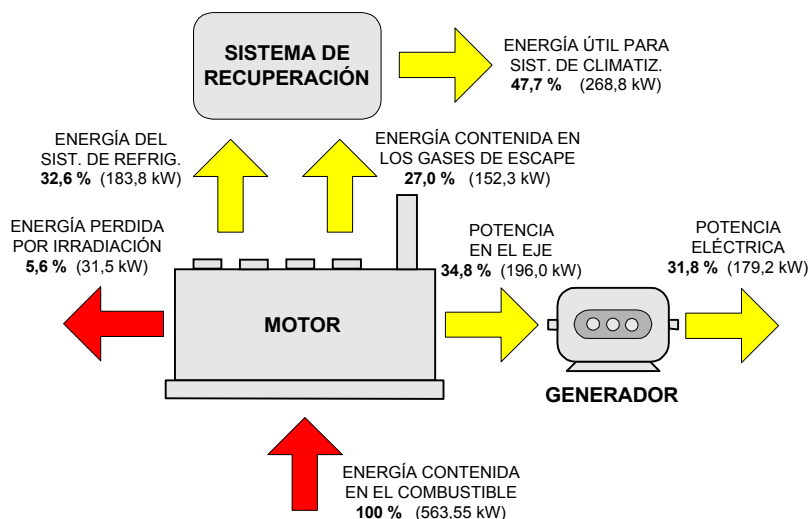
Figura 1. Potencias involucradas
