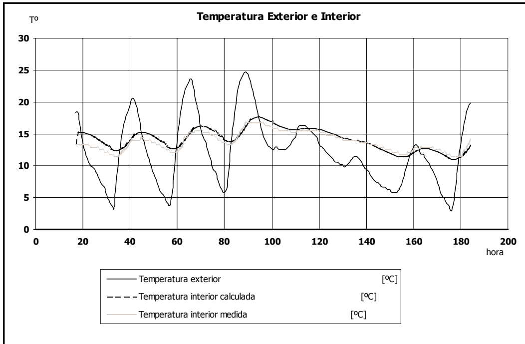
Figura 2: Gráfico de temperaturas para una vivienda del Barrio Santa Lucia, Provincia de San Juan. Las temperaturas exteriores fueron medidas in situ y las interiores una medida y otra obtenida mediante la simulación.
